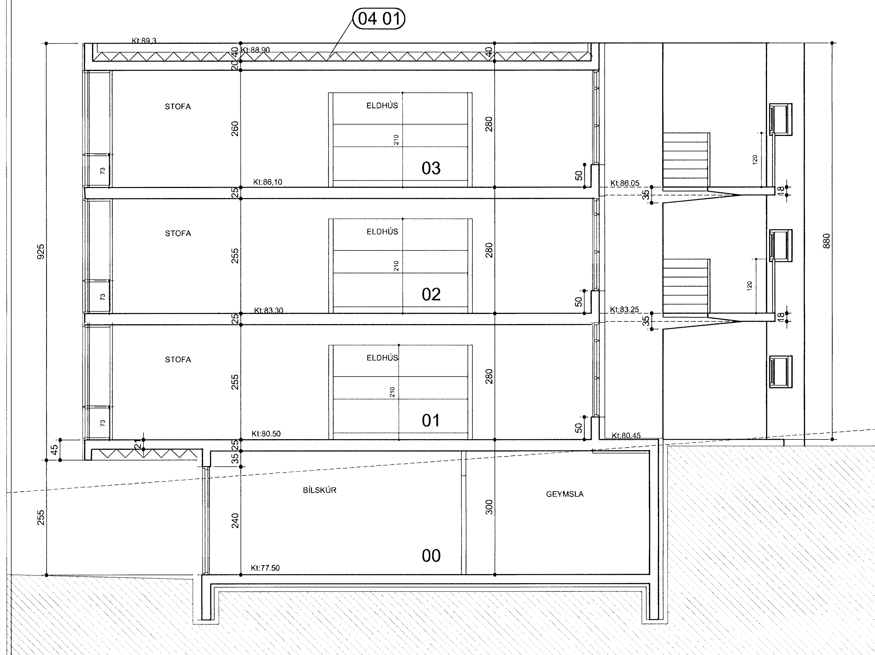
SNEIÐING A-A
