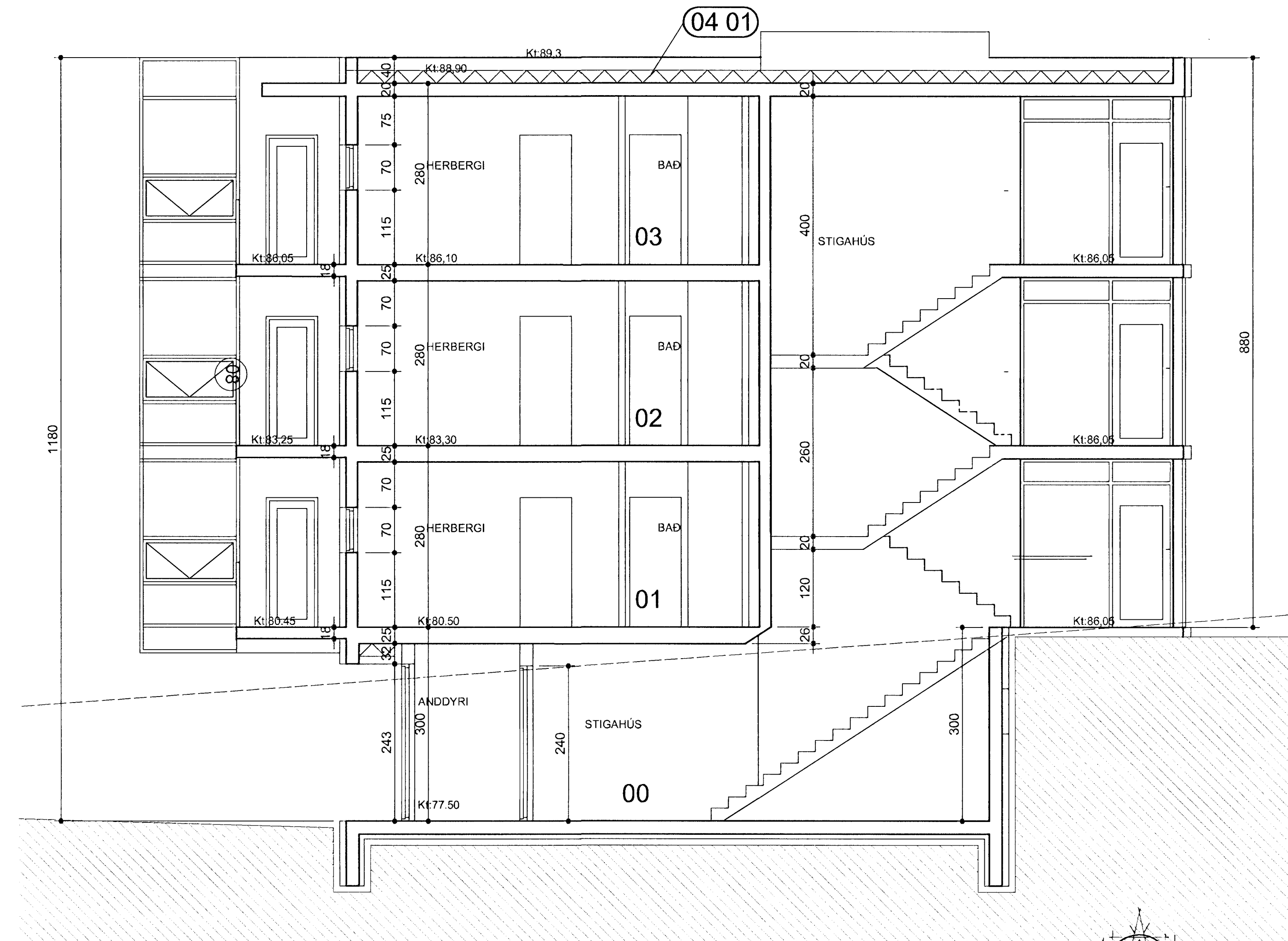
SNEIÐING B-B
