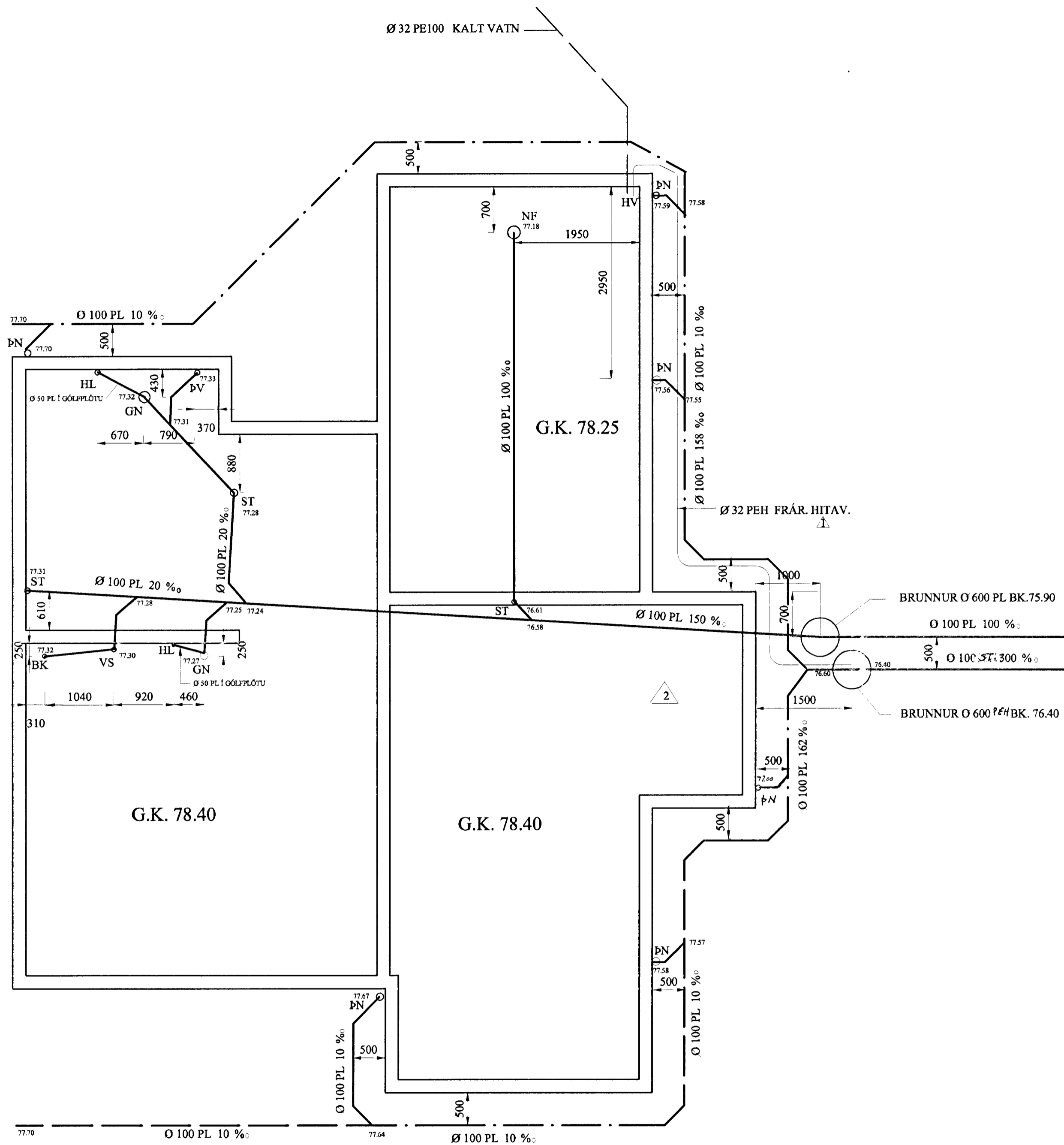
ERLUÁS 36 GRUNNMYND 1:50
