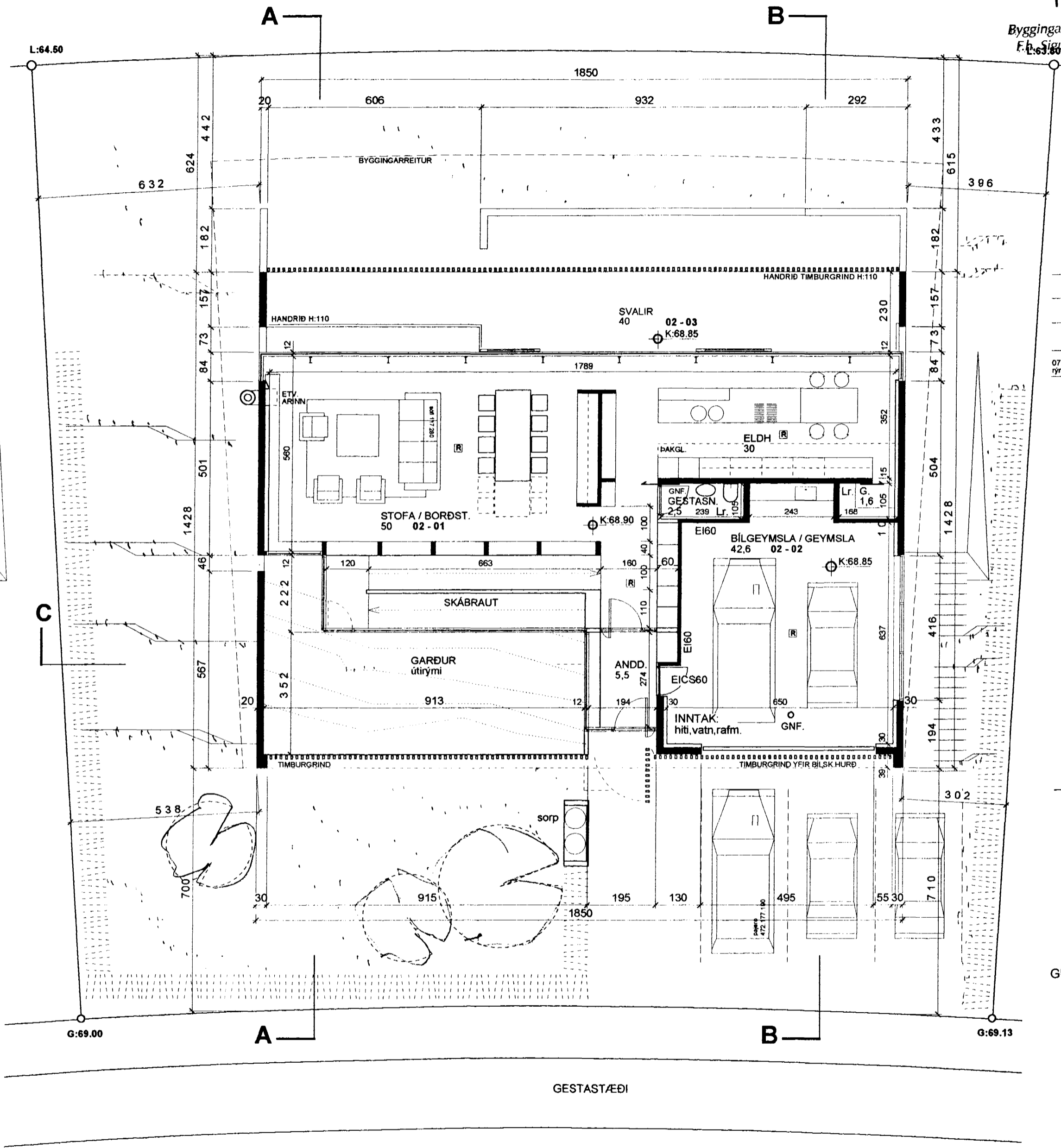
GRUNNMYND EFRI HÆÐAR MKV. 1:100
