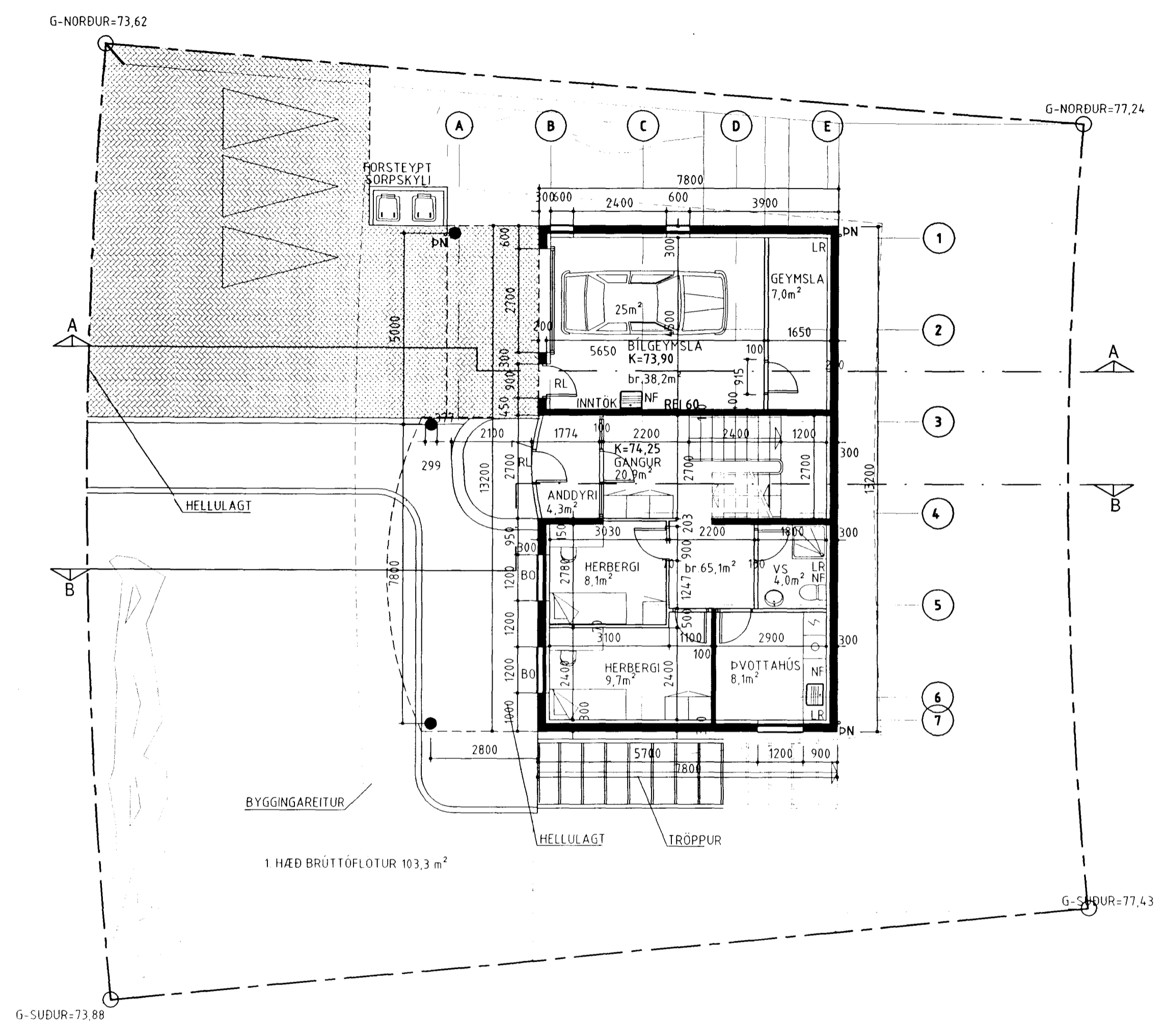
GRUNNMYND 1. HÆÐAR 1:100
