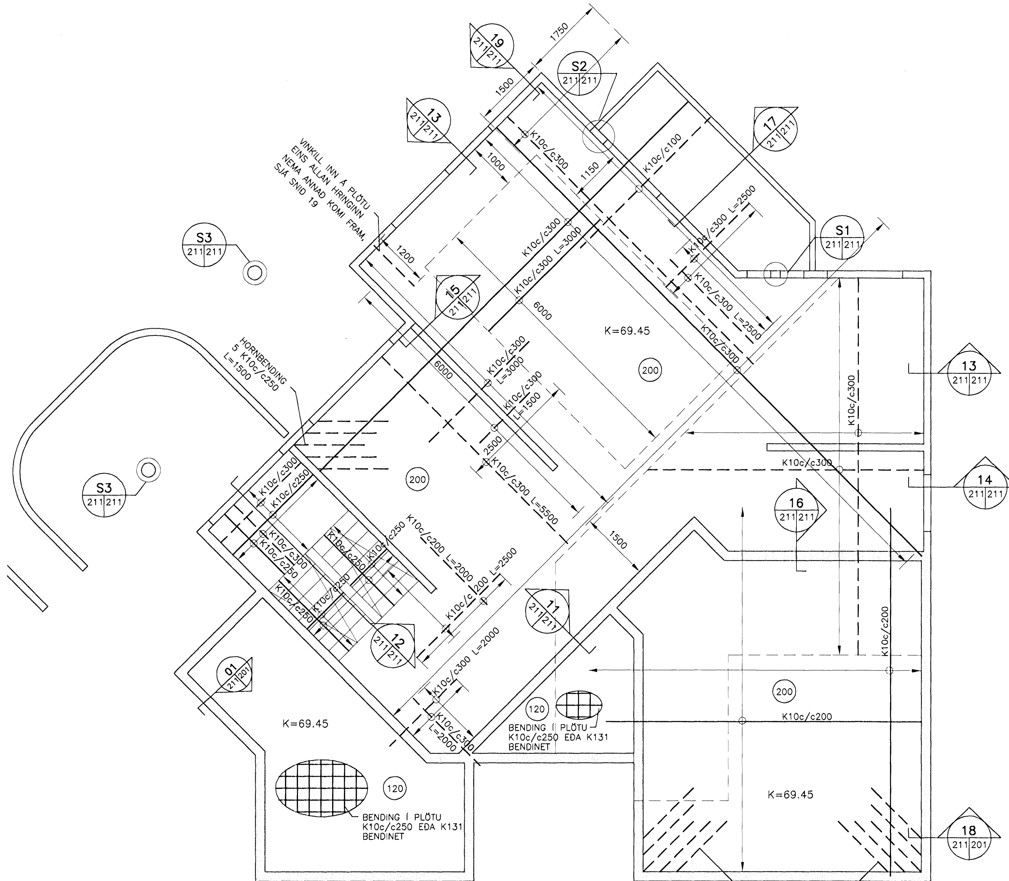
GRUNNMYND, 1:50
