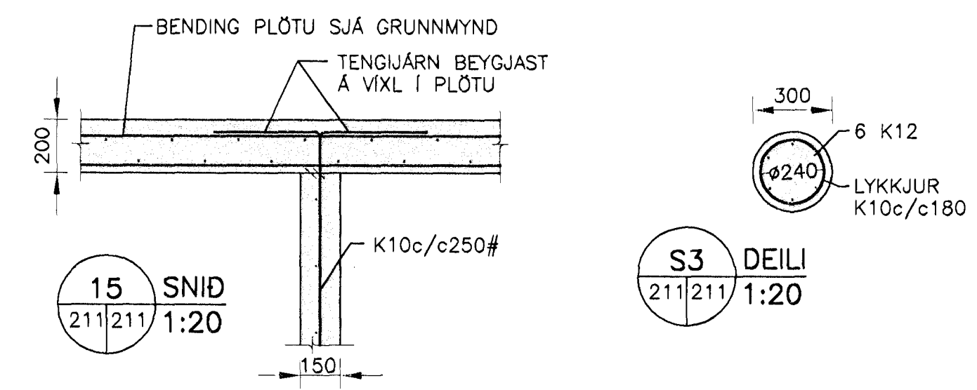
11 SNID 211|211 1:20
