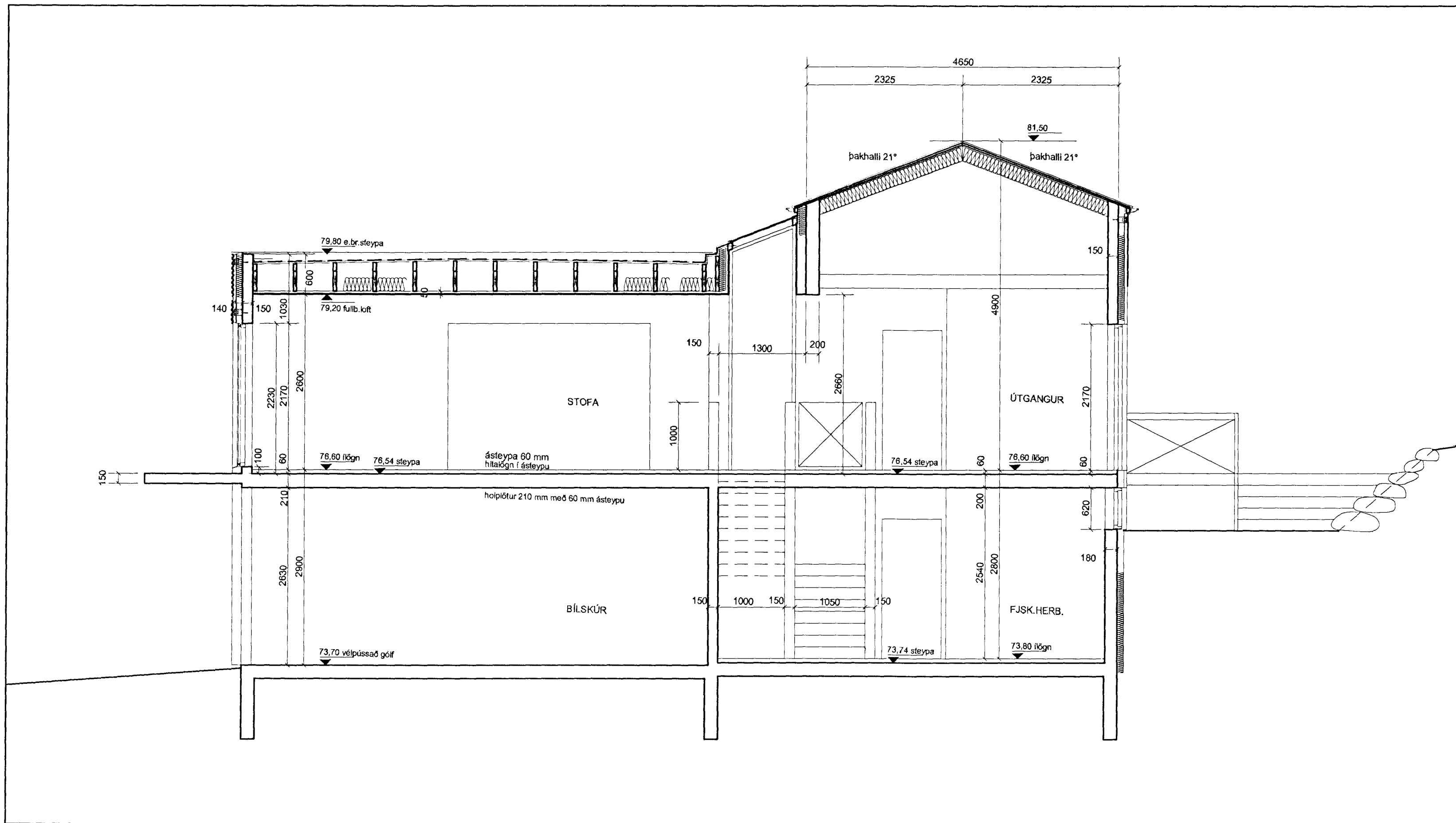
snið A - A, m = 1:50
