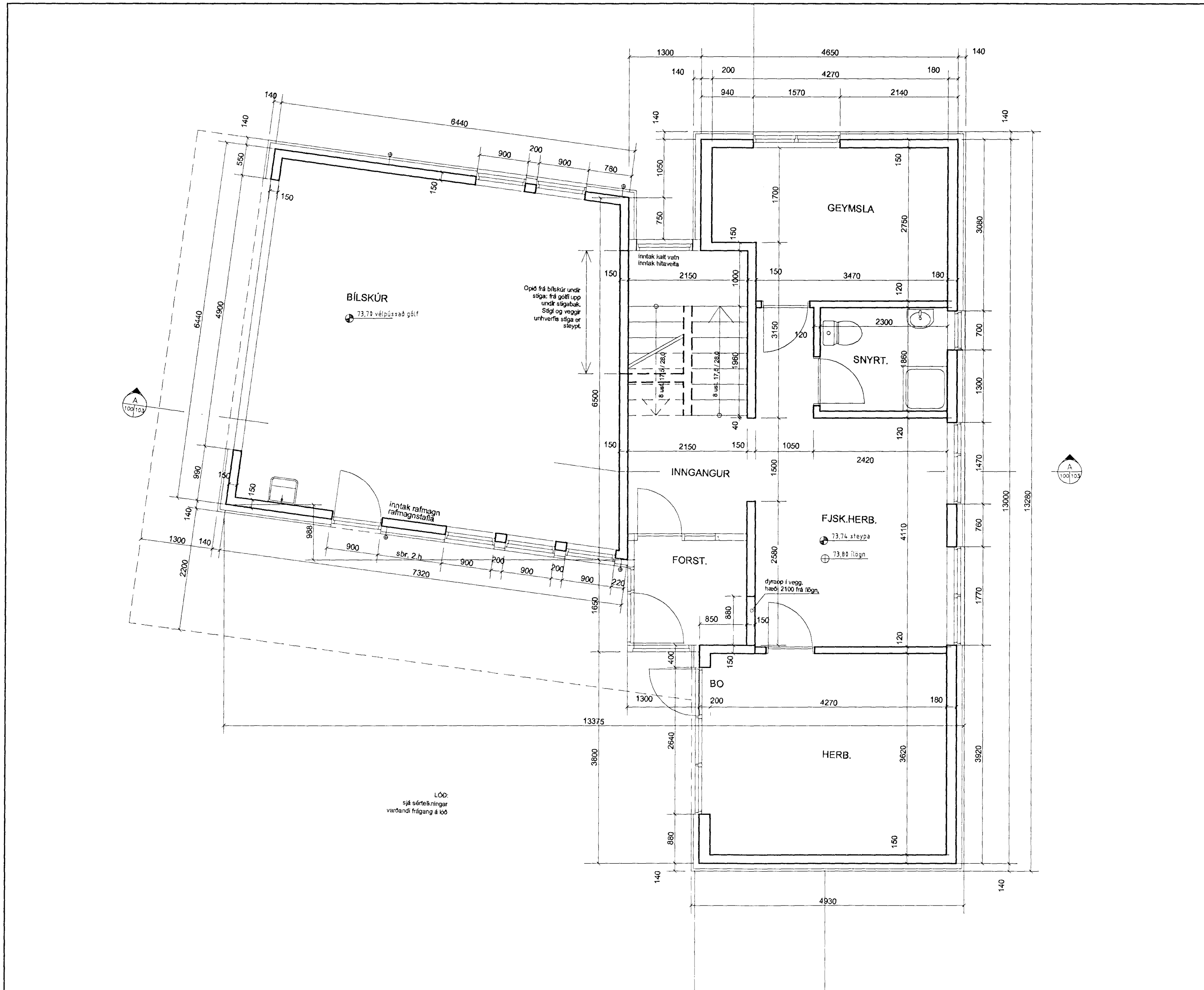
GRUNNMYND 1. hæð m = 1:50
