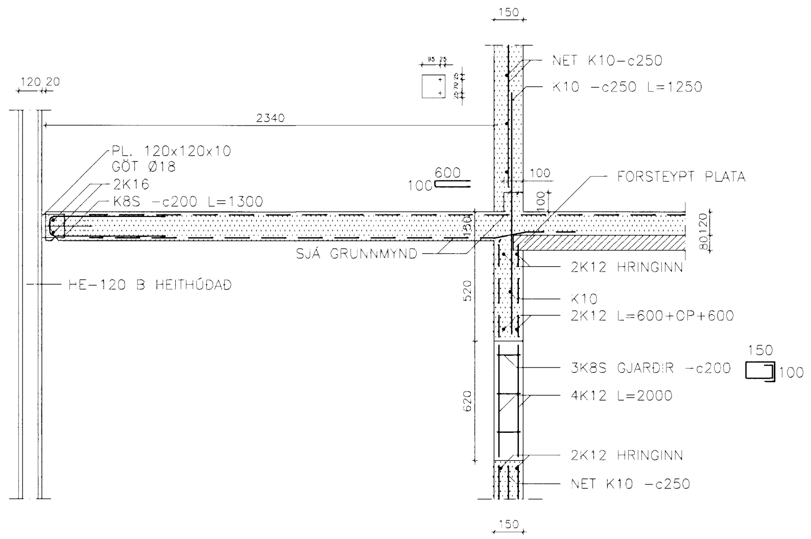
SNID 14-14 MKV. 1:20
