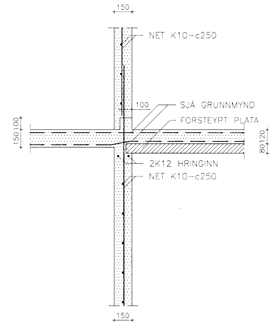
SNID 15-15 MKV. 1:20
