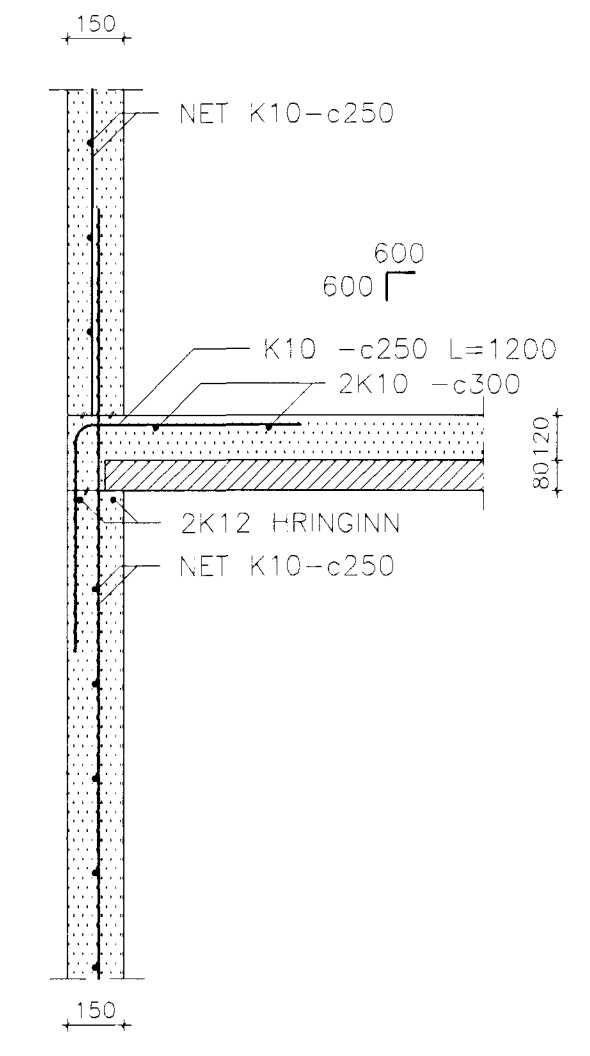
SNID 16-16 MKV. 1:20
