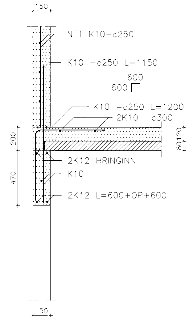
SNID 17-17 MKV. 1:20
