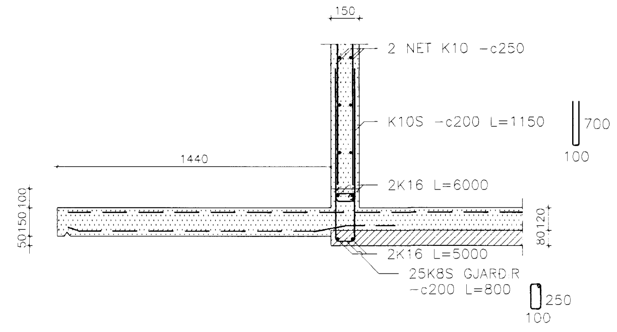
SNID 19-19 MKV. 1:20
