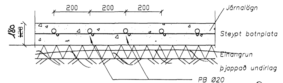
Gölfhiti þversnið 1:10
