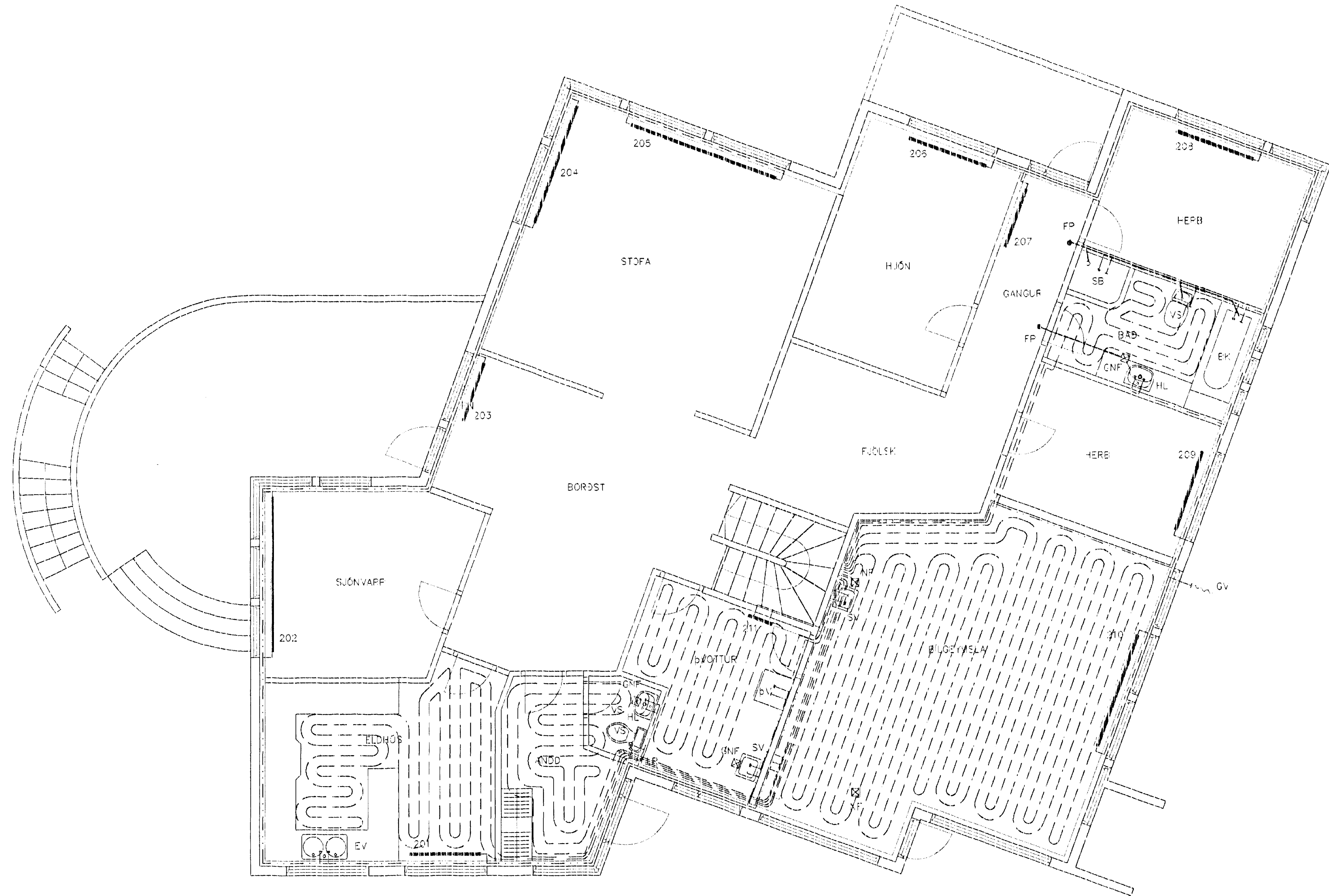
GRUNNMYND 2. HÆÐAR 1:50
