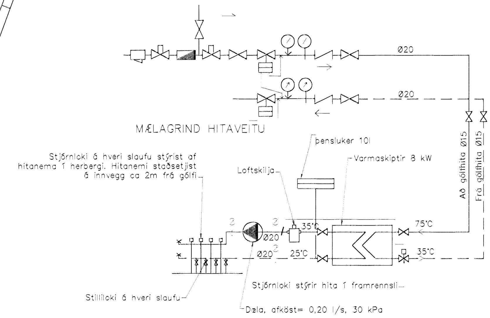
TENING GÓLFHITA
