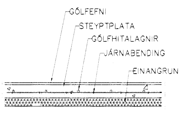
GÓLFHITI SNIÐ, 1:20
