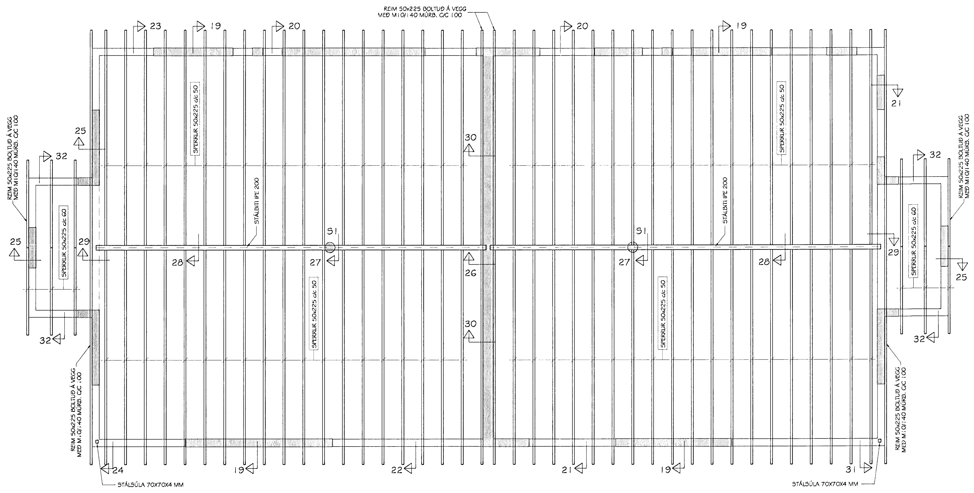
GRUNNMYND ÞAKVIÐA MKV. 1:50
