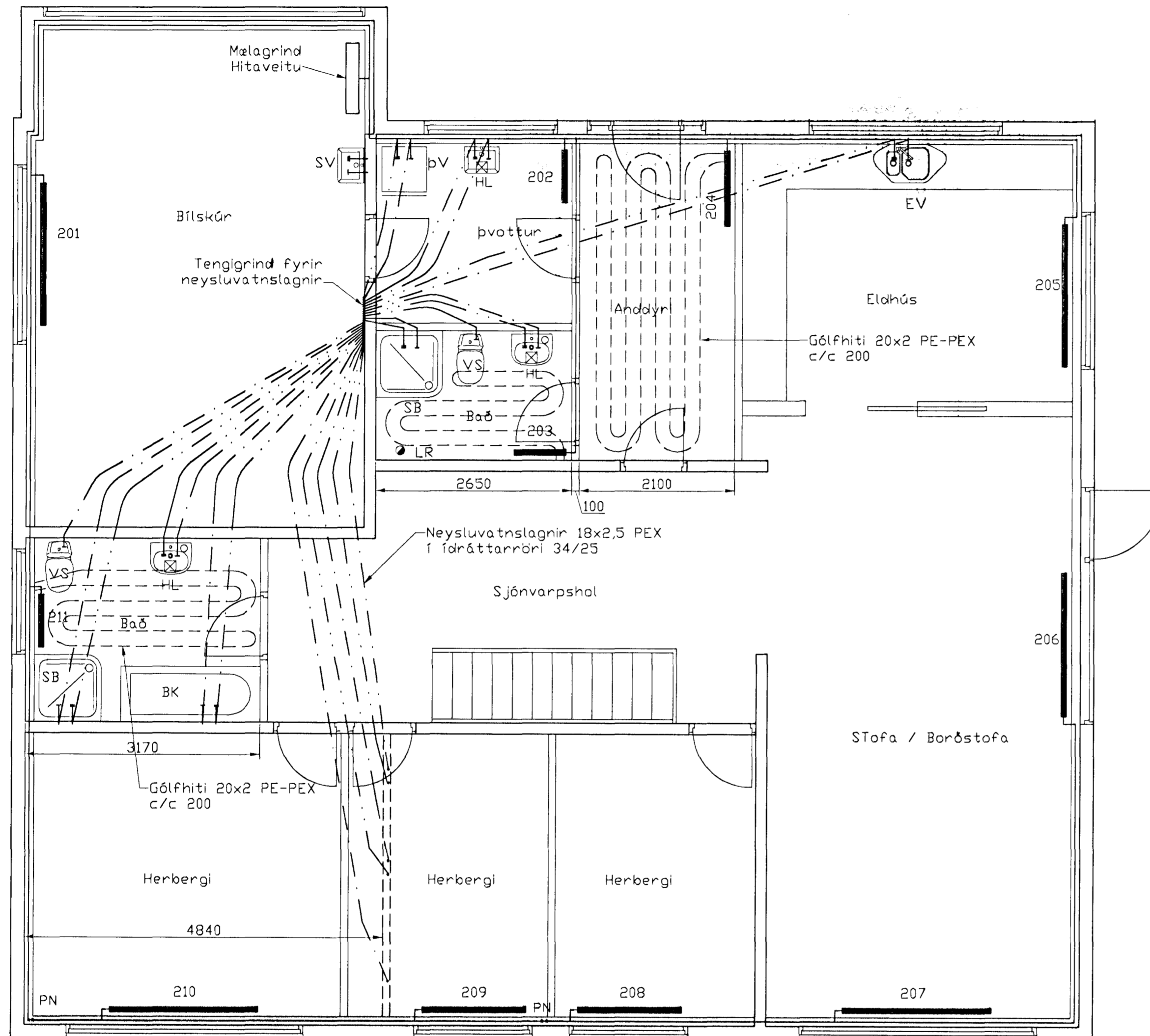
2. hæð, Grunnmynd, 1:50
