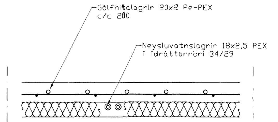
Gólfagnir, Snið 1:10
