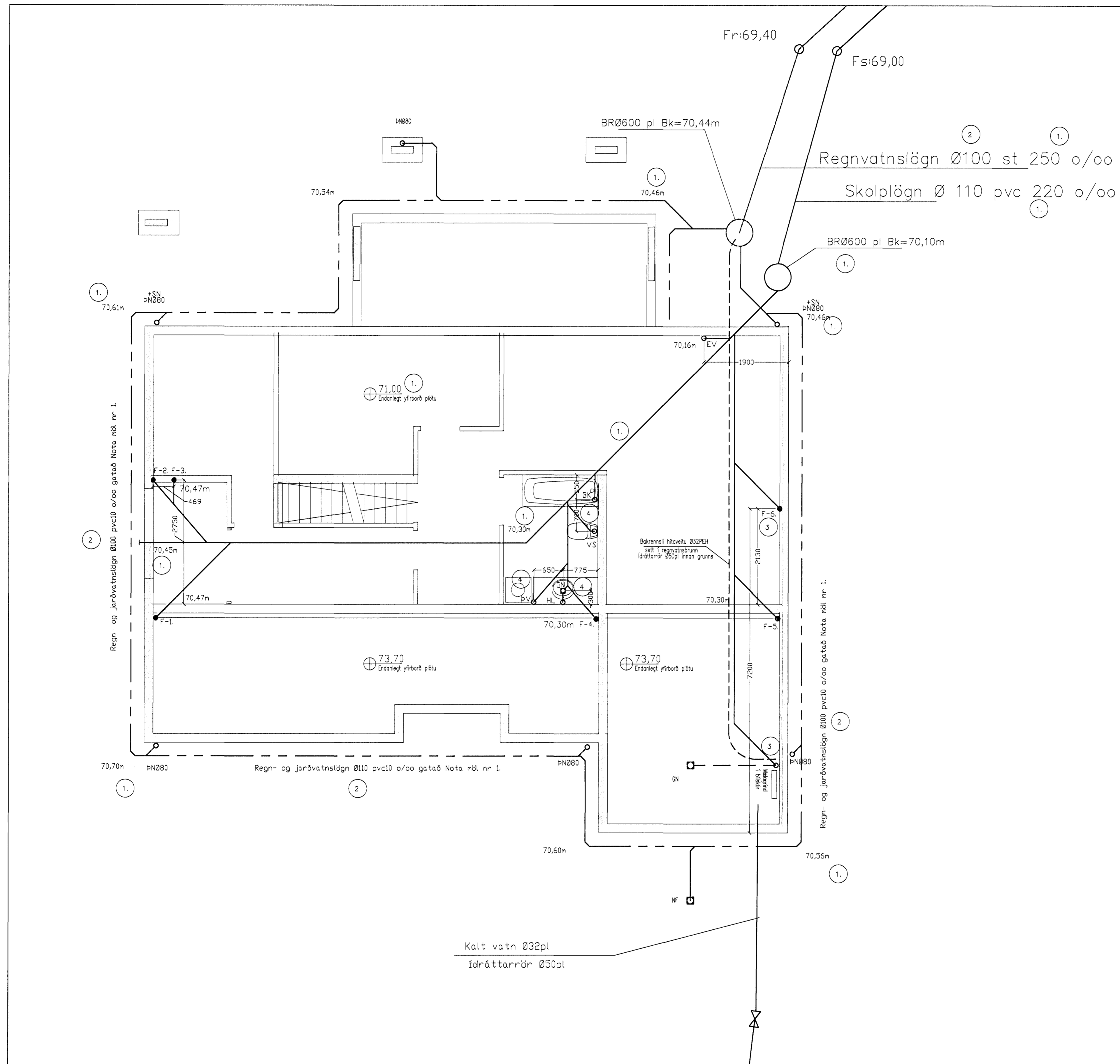
Grunnmynd 1.50.
