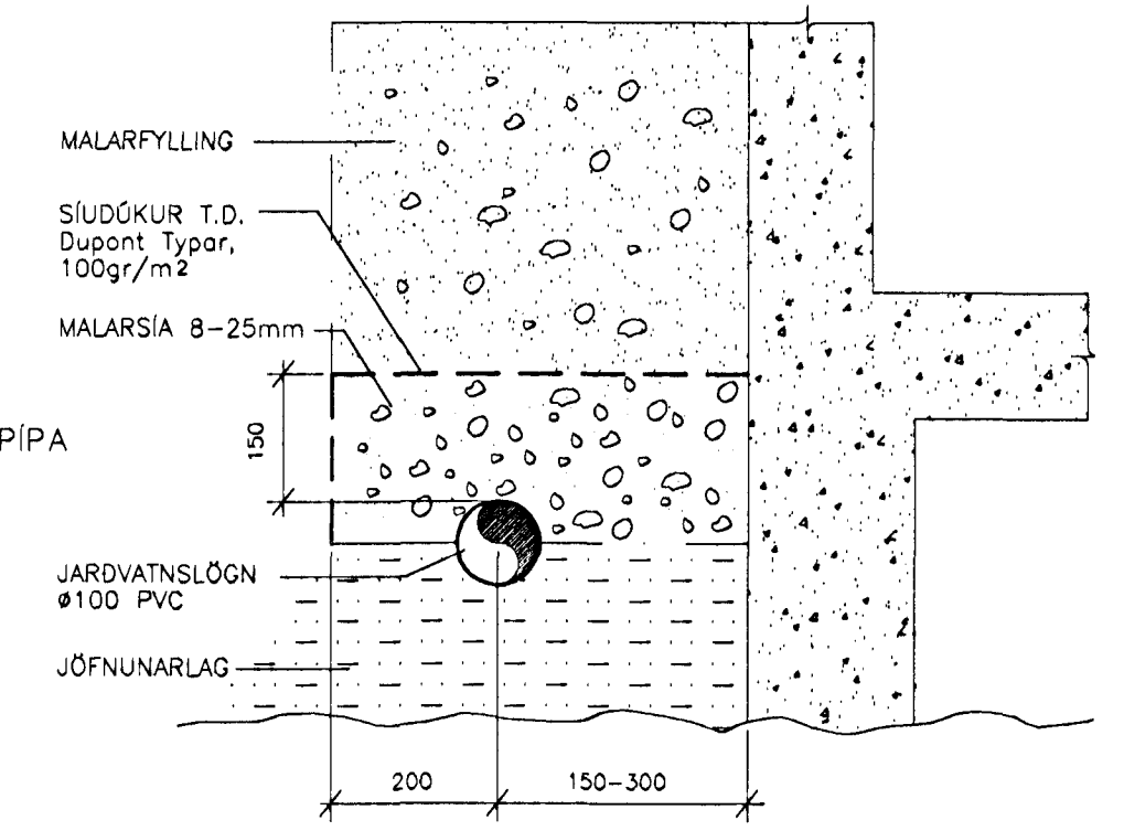
FRÁGANGUR JARÐVATNSLAGNA ÓR PVC M=1:20
