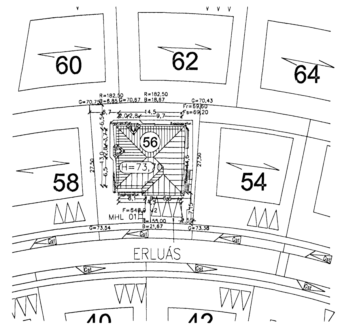
AFSTÖÐUMYND 1:500
