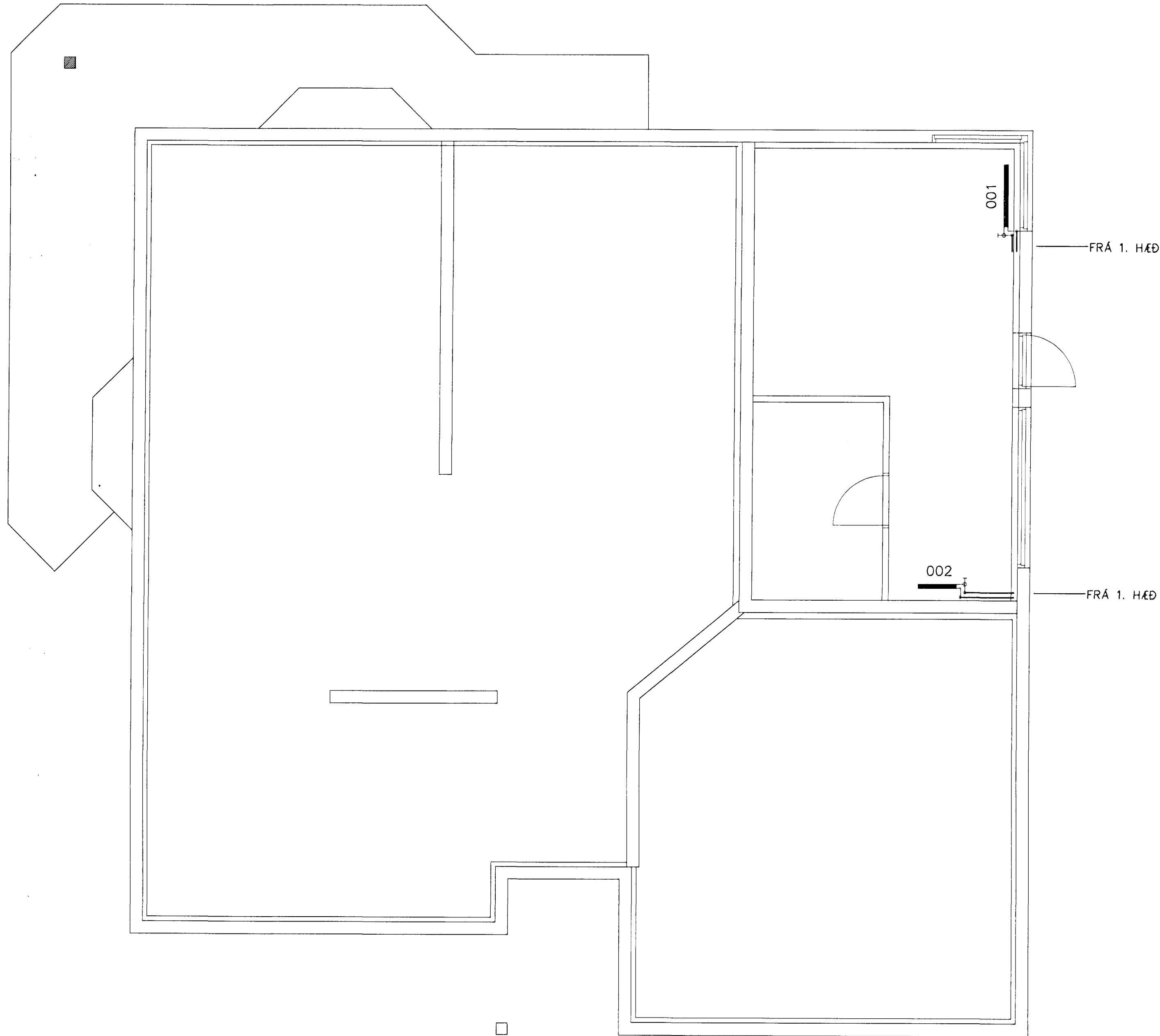
GRUNNMYND 1:50
