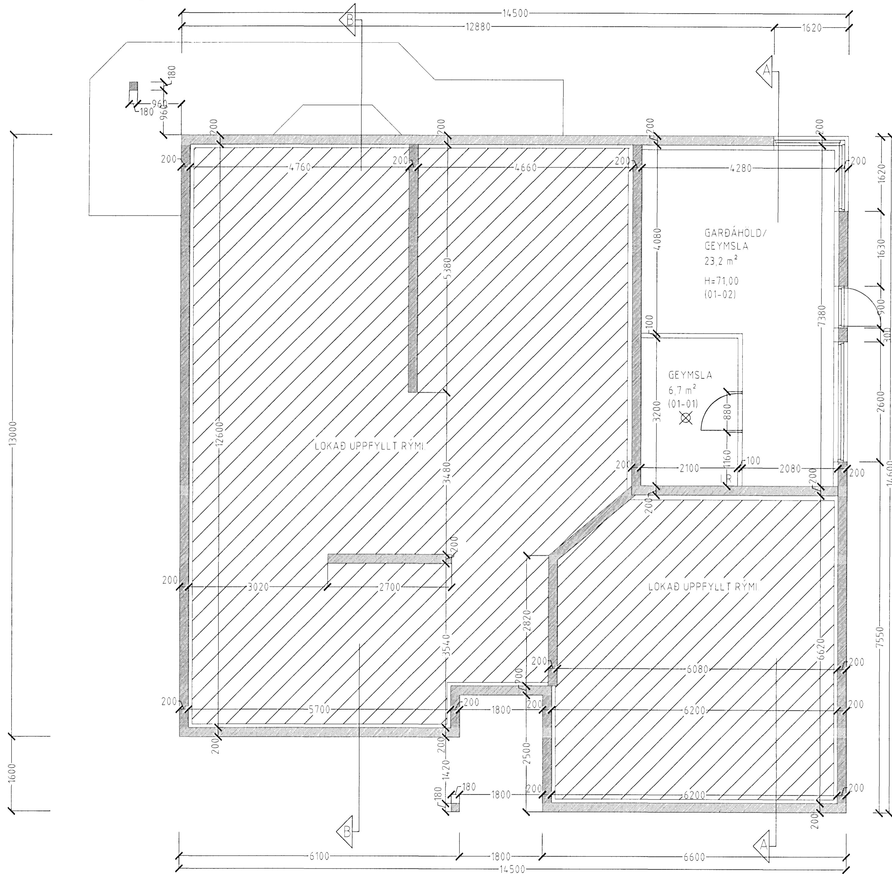
GRUNNMYND JARÐHÆÐ MKV. 1:50.
