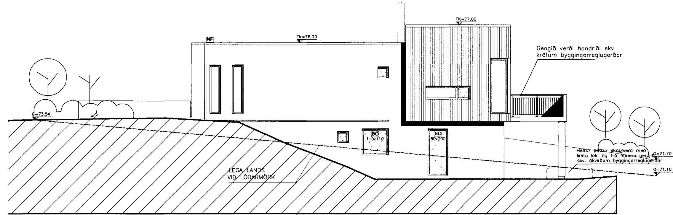
ÚTLIT NORDUR
