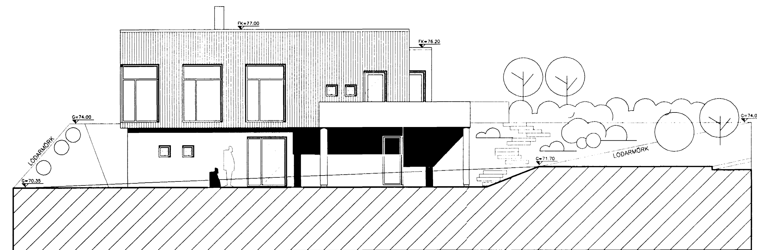
ÚTLIT VESTUR
