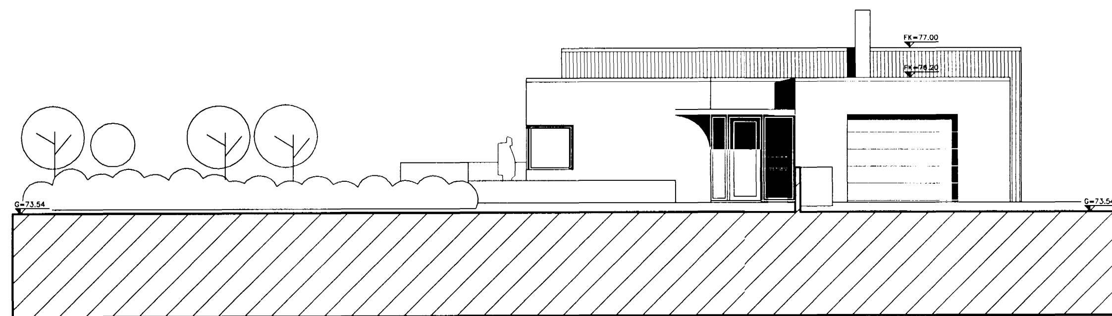
ÚTLIT AUSTUR
