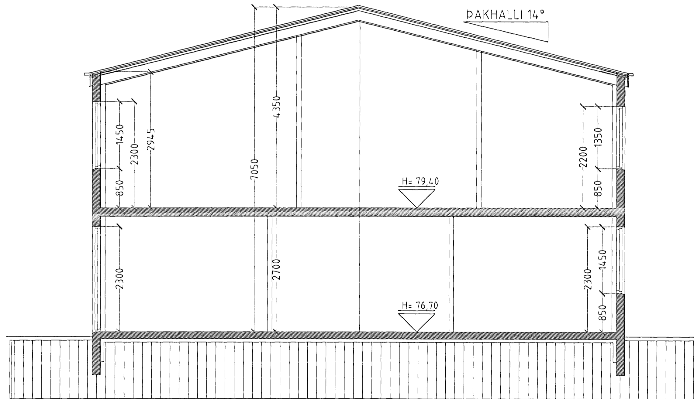
SNID A - A M. 1:50
