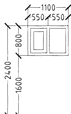
2 STK. BIFREIDAGEYMSLA.
