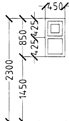
2 STK. BAÐ.
