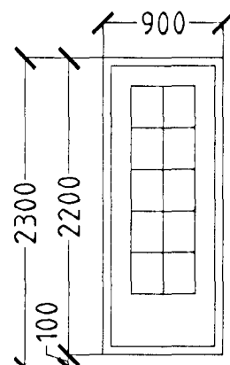
1 STK. FJÖLSKYLDA. HURÐ OPNAST HÆGRI ÚT.
