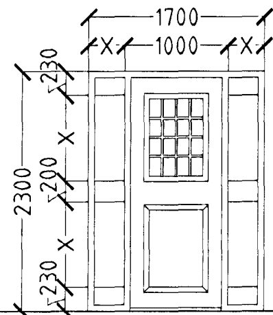
1 STK. ANDDYRI HURÐ OPNAST HÆGRI ÚT.
