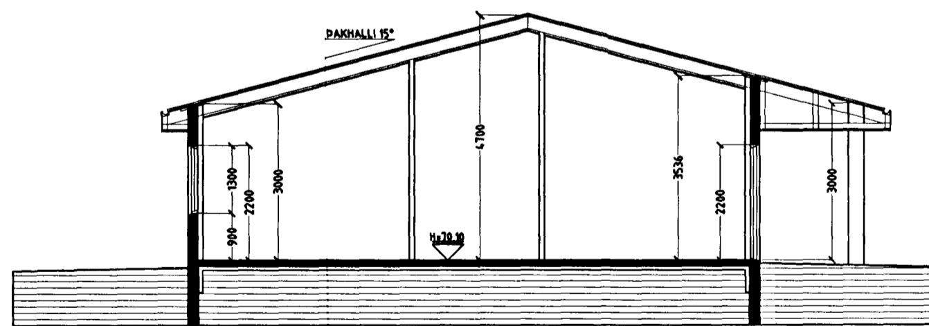
SNID B-B MKV. 1:100.
