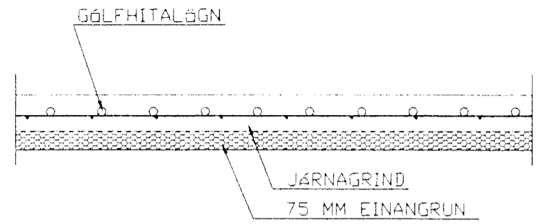
SNID 1 GÖLFHITALAGN 1:20
