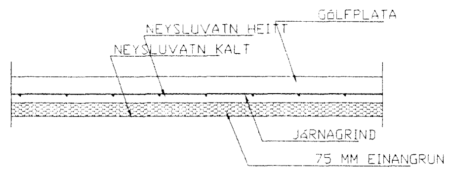
SNID Í NEYSLUVATN Í GÖLFI 1:20 RÖR Í RÖR EINANGRAST MEÐ EINANGRUNARHÖLKUM
