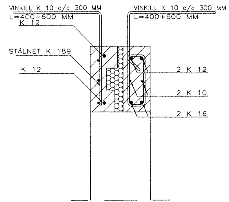
SNID -G 1:10
