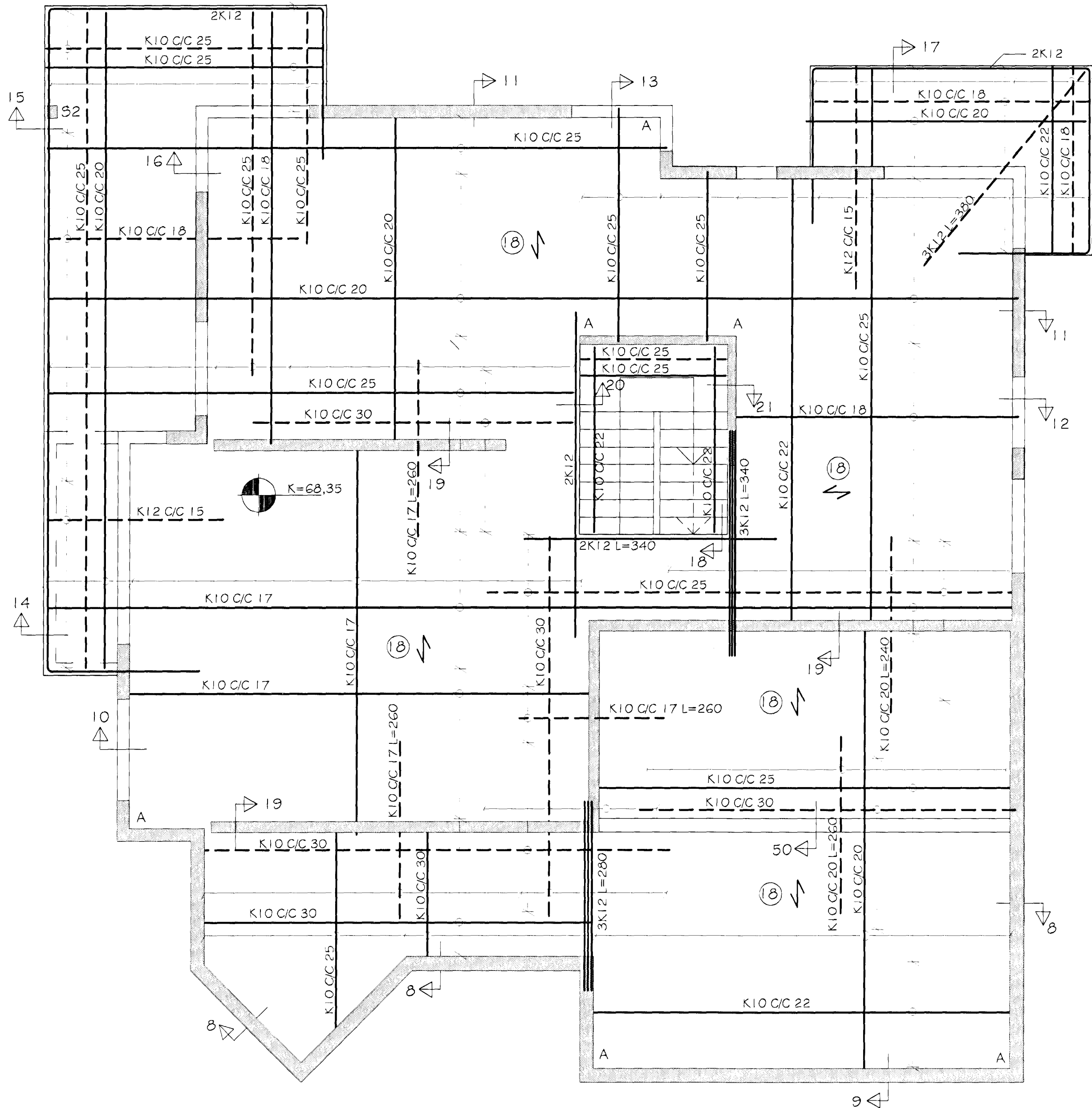
JÁRN Í PLÖTU YFIR NEÐRI HÆÐ GRUNNMYND MKV. 1:50
