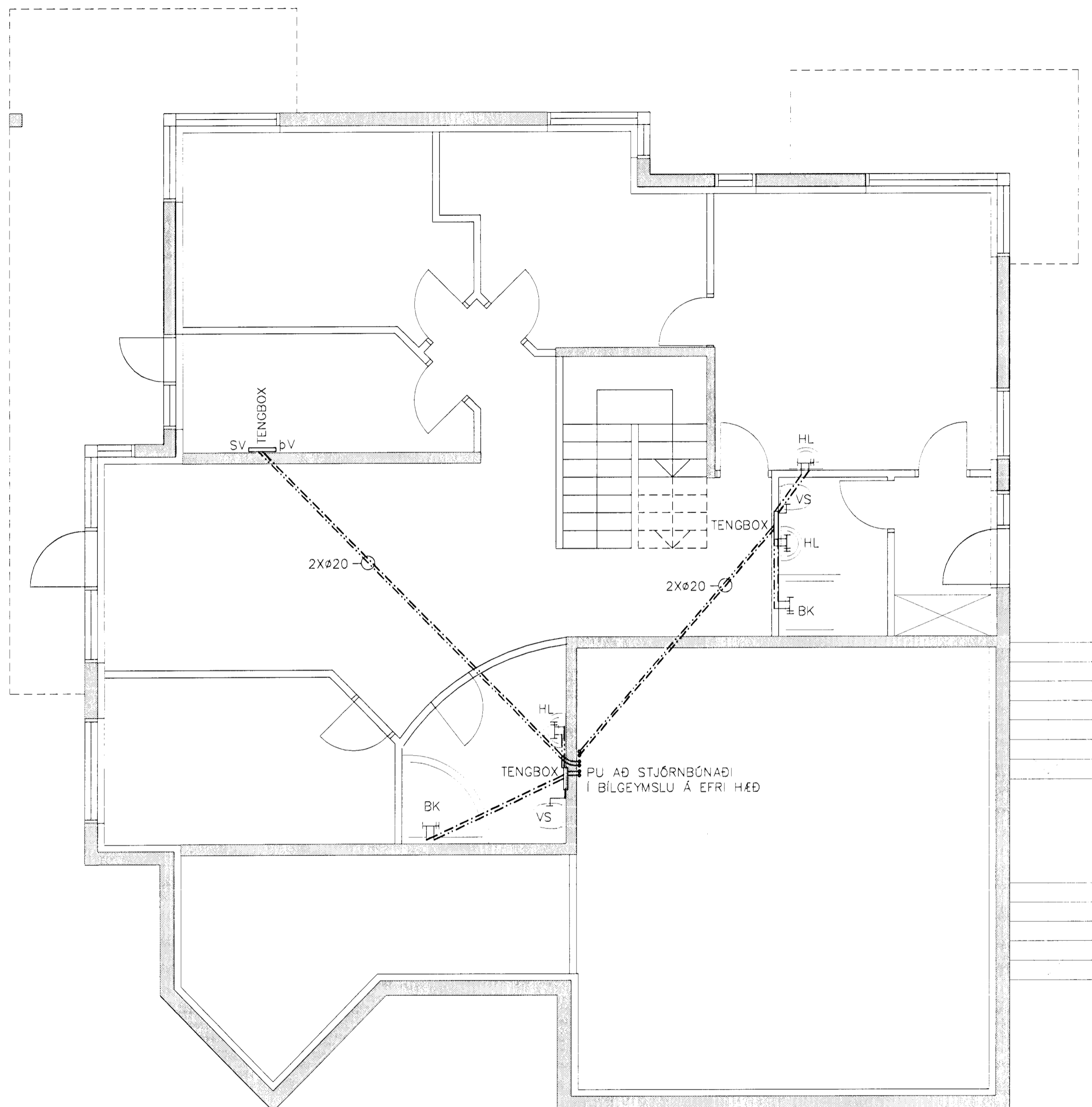
NEYSLUVATNSLAGNIR GRUNNMYND NEDRI HÆÐAR MKV. 1:50
