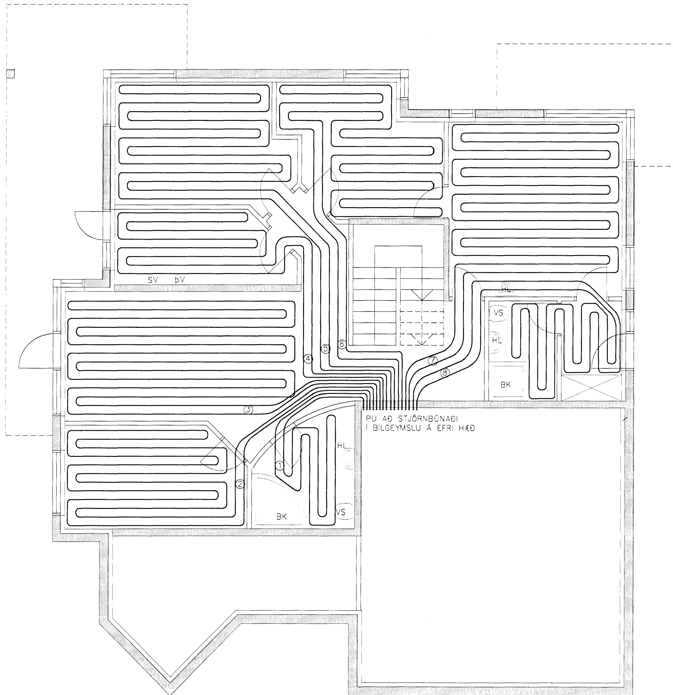
HITALAGNIR GRUNNMYND NEDRI HÆÐAR MKV. 1:50
