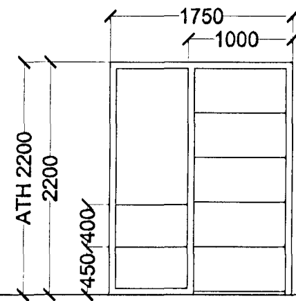
1 STK. ANDDYRI. HURÐ OPNAST HÆGRI ÚT.
