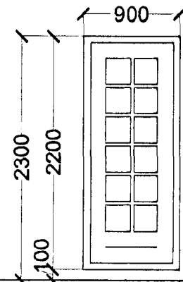
1 STK. FJÖLSKYLDA. HURÐ OPNAST HÆGRI ÚT.
