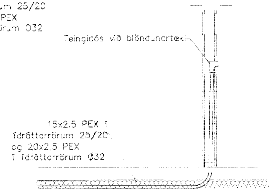
TENING NEYSLUVATNSLAGNA 1:20
