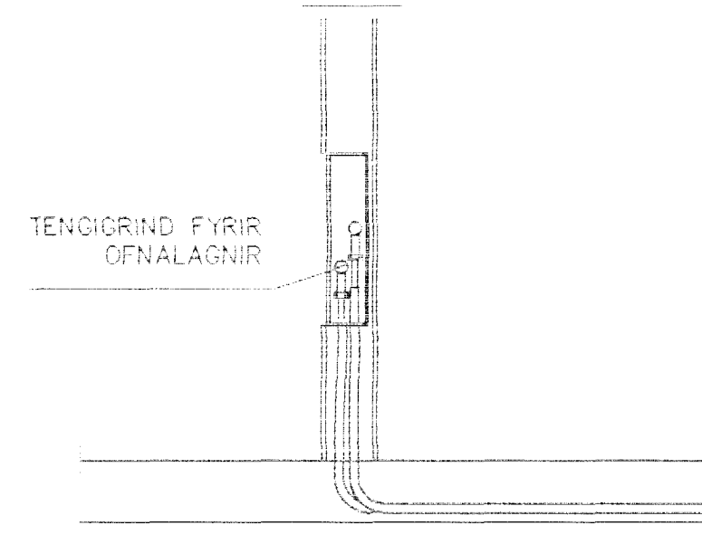
TENING OFNALAGNA 1:20
