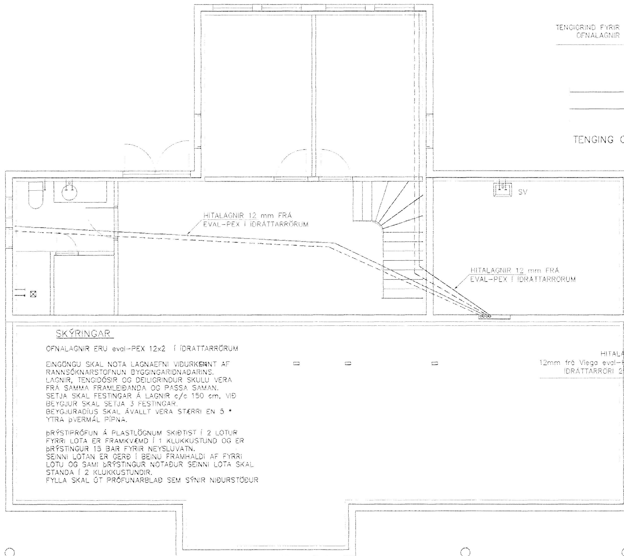
GRUNNMYND 1 HÆÐAR 1:50
