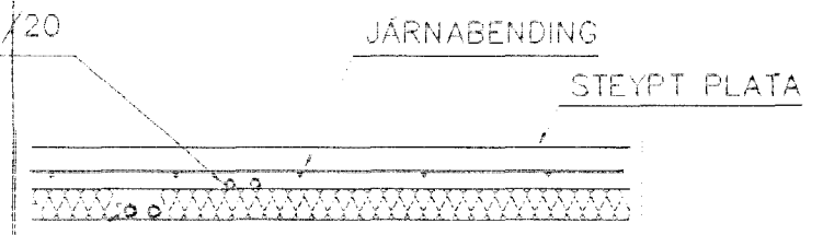
LAGNIR, SNIÐ, 1:20
