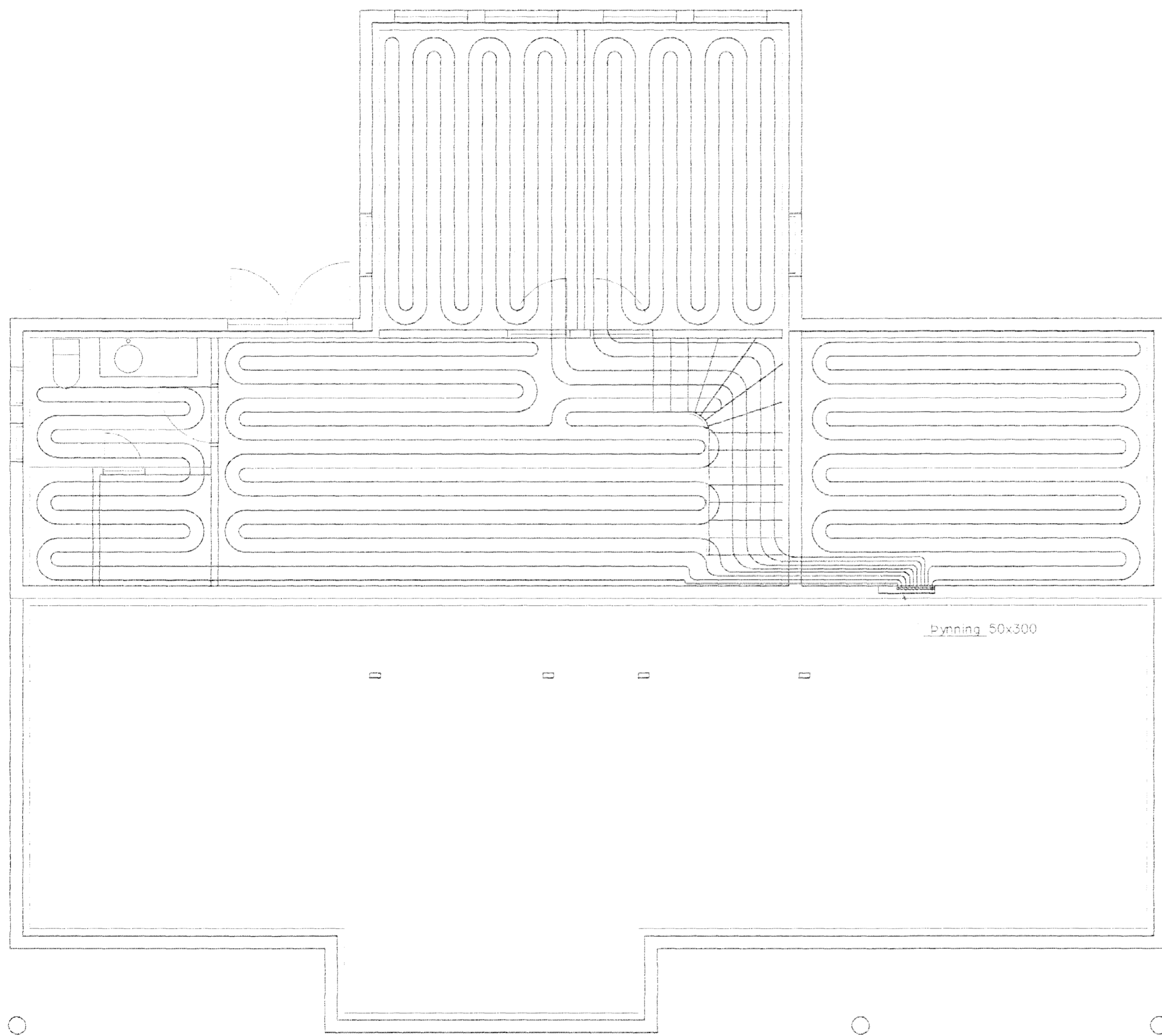
GRUNNMYND 1 HÆÐAR 1:50
