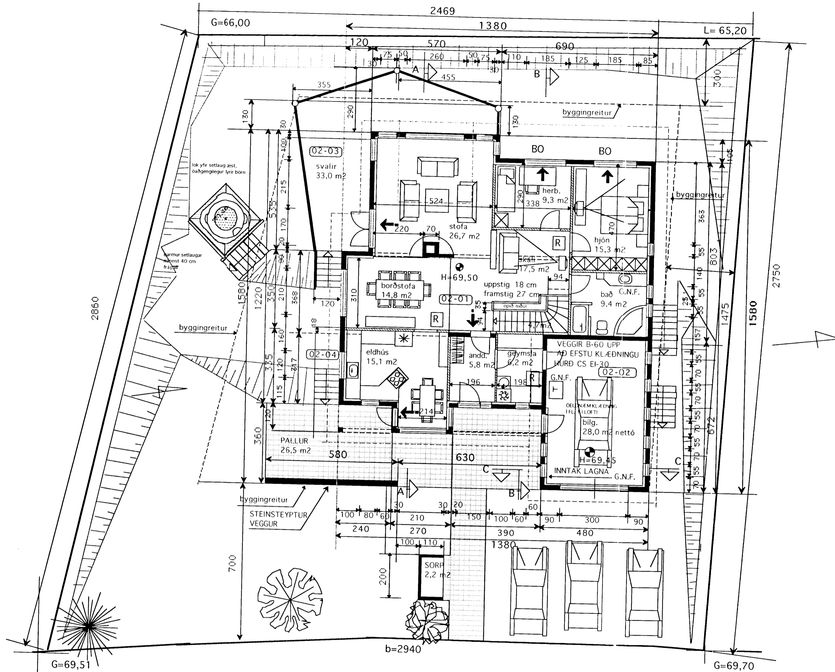
G=69,51 GRUNNMYND 2 HÆÐ 1:100 Nánari málsetning sjá teikn.V-1 1:50
