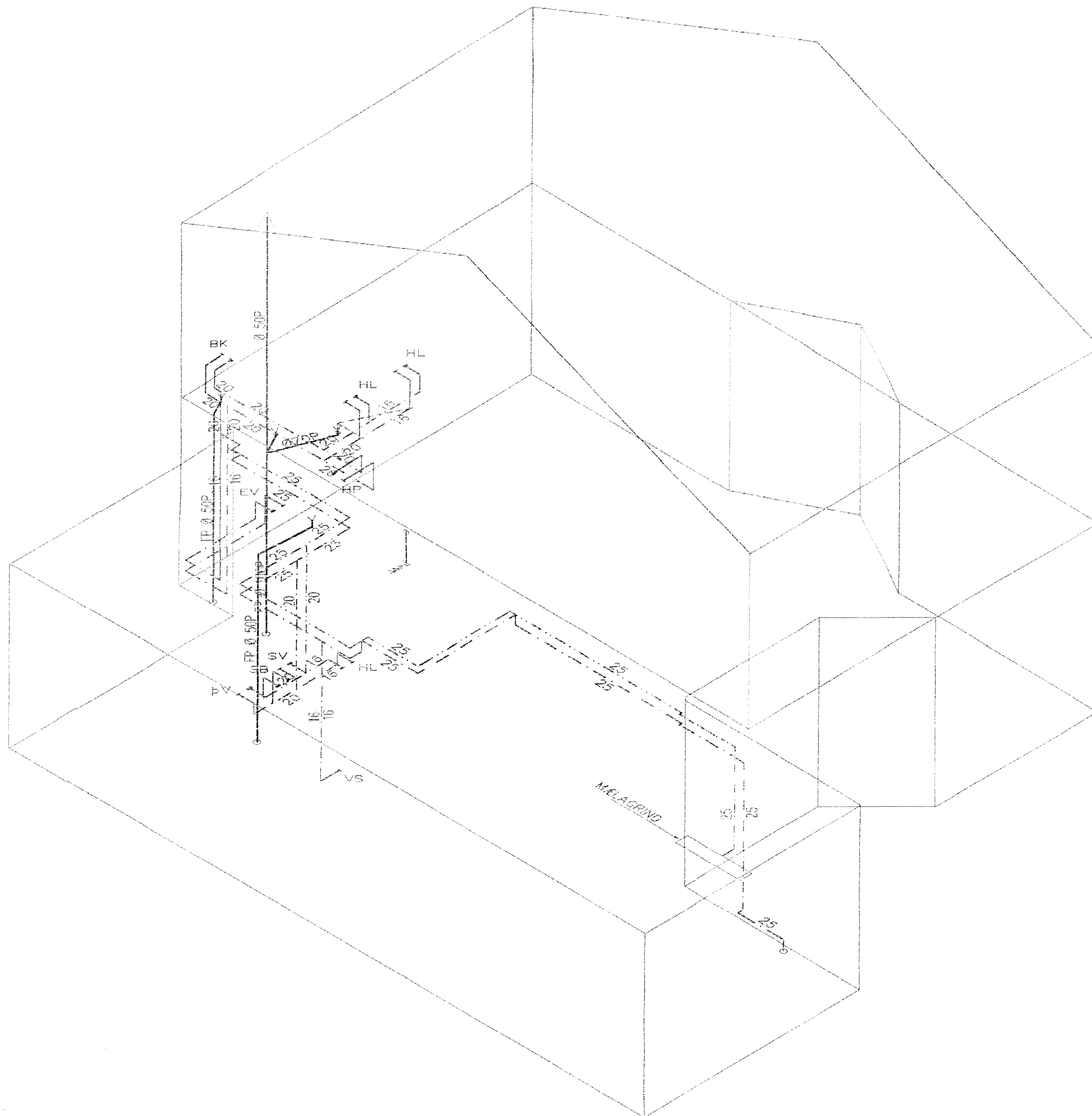
RÖMMYND VATNSLAGNA 1:50
