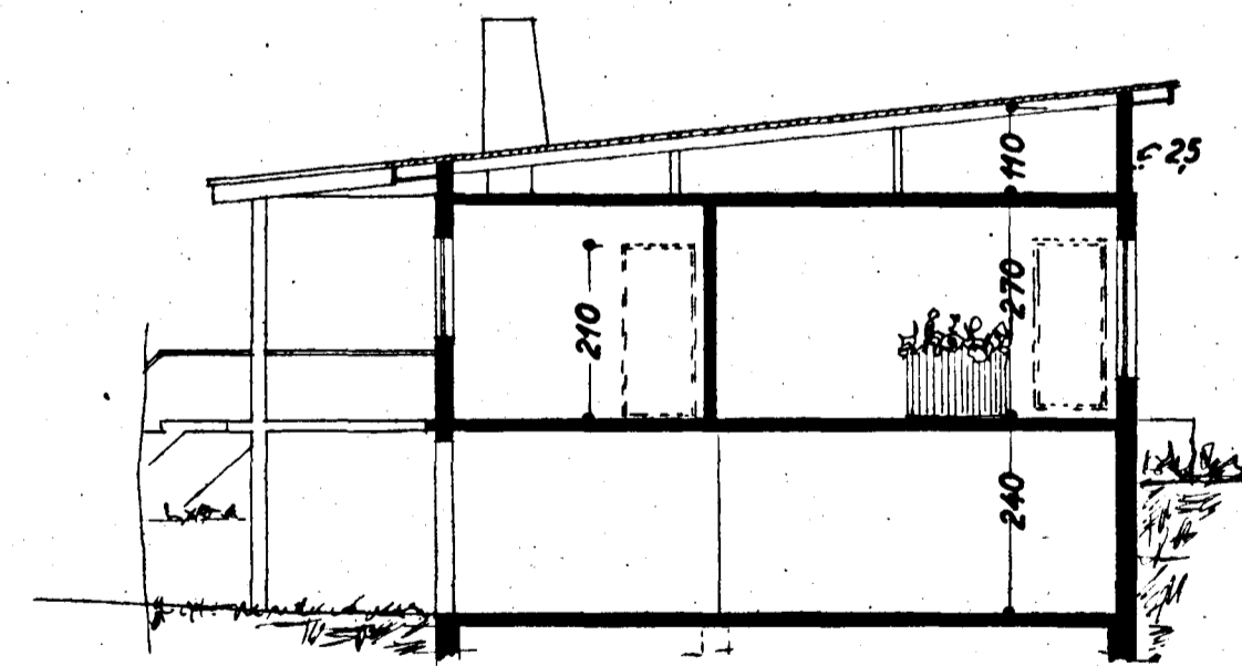
Snið A-A
