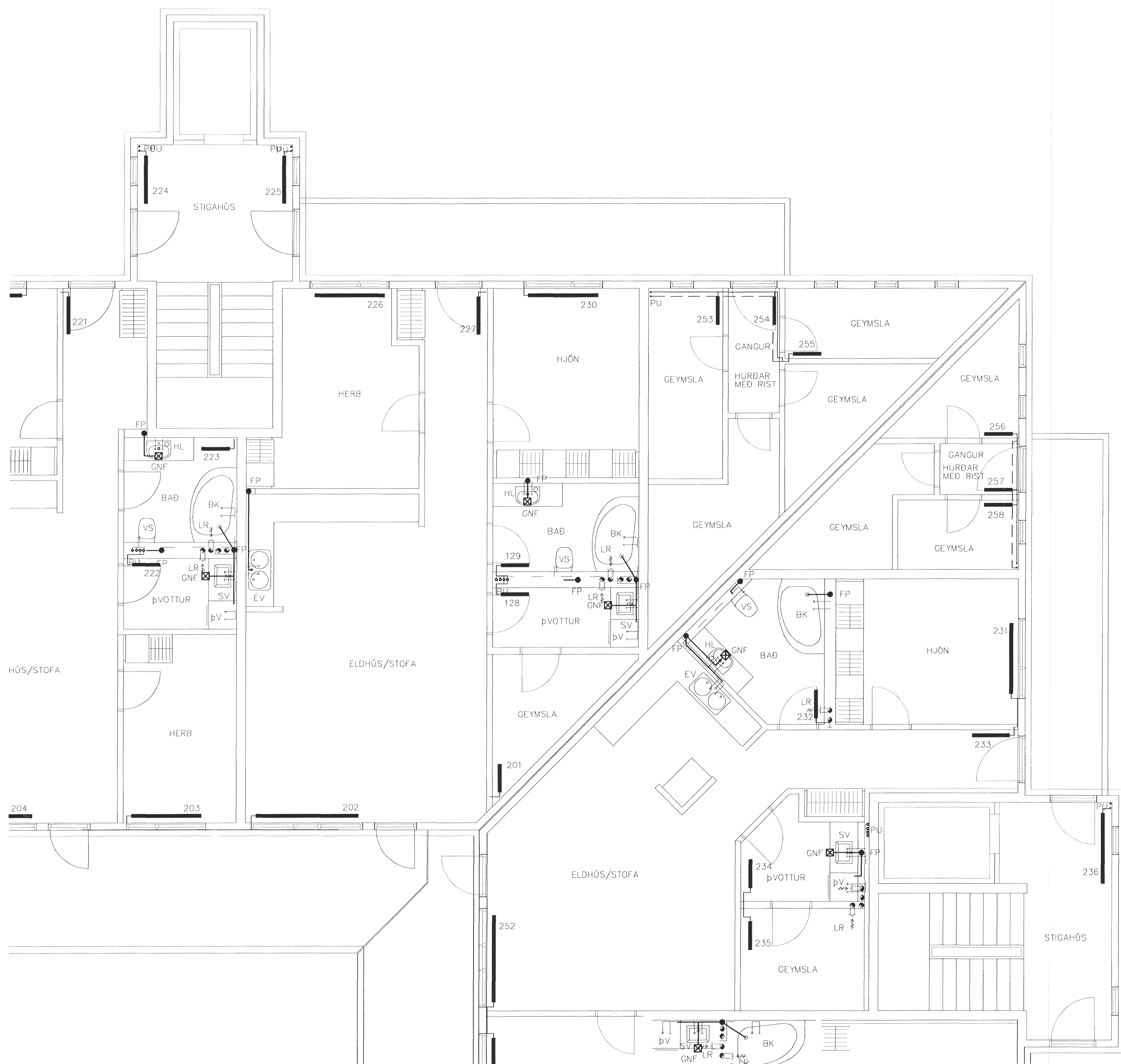
GRUNNMYND 2 HÆÐAR 1:50
