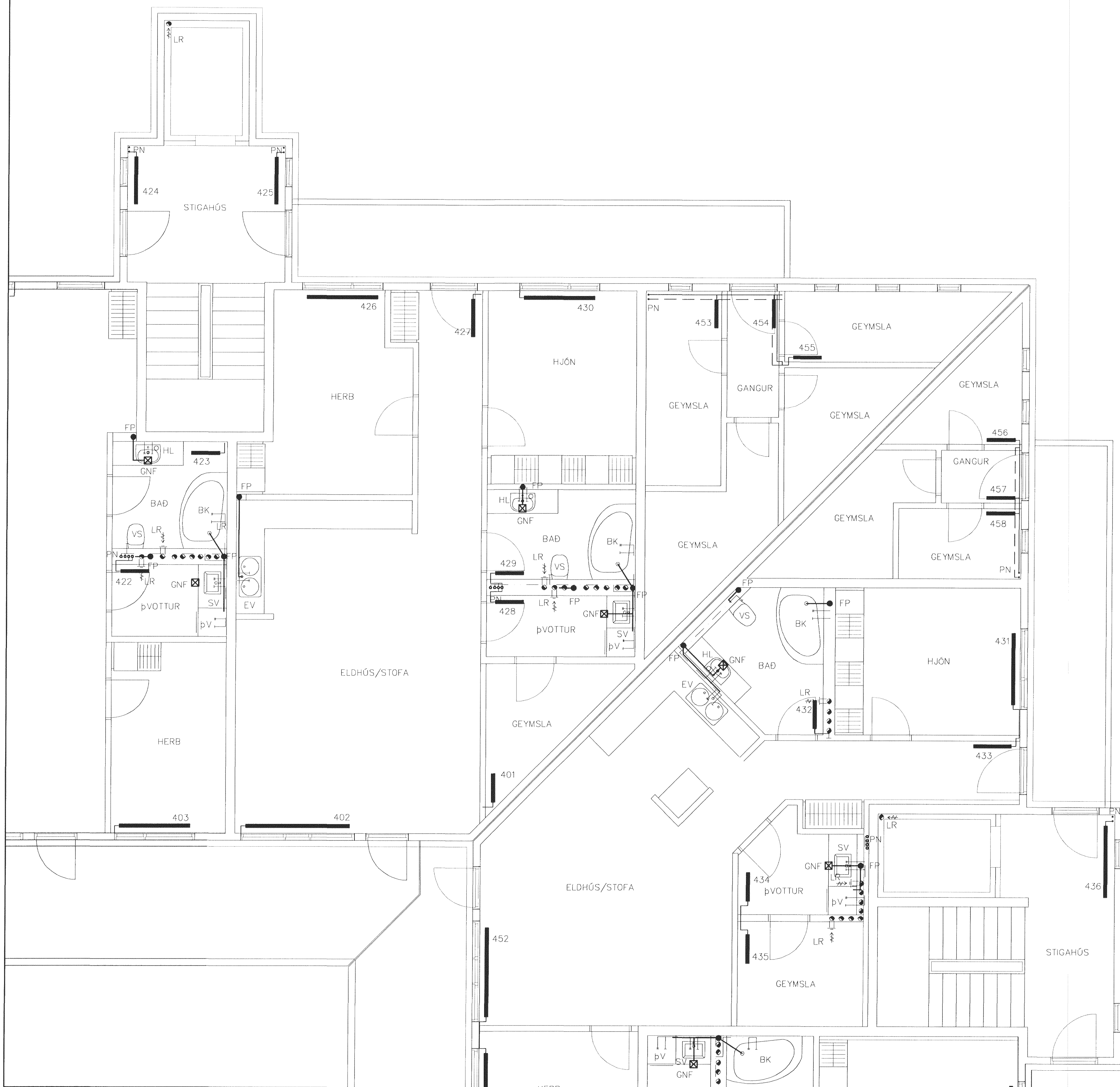
GRUNNMYND 4 HÆÐAR 1:50
