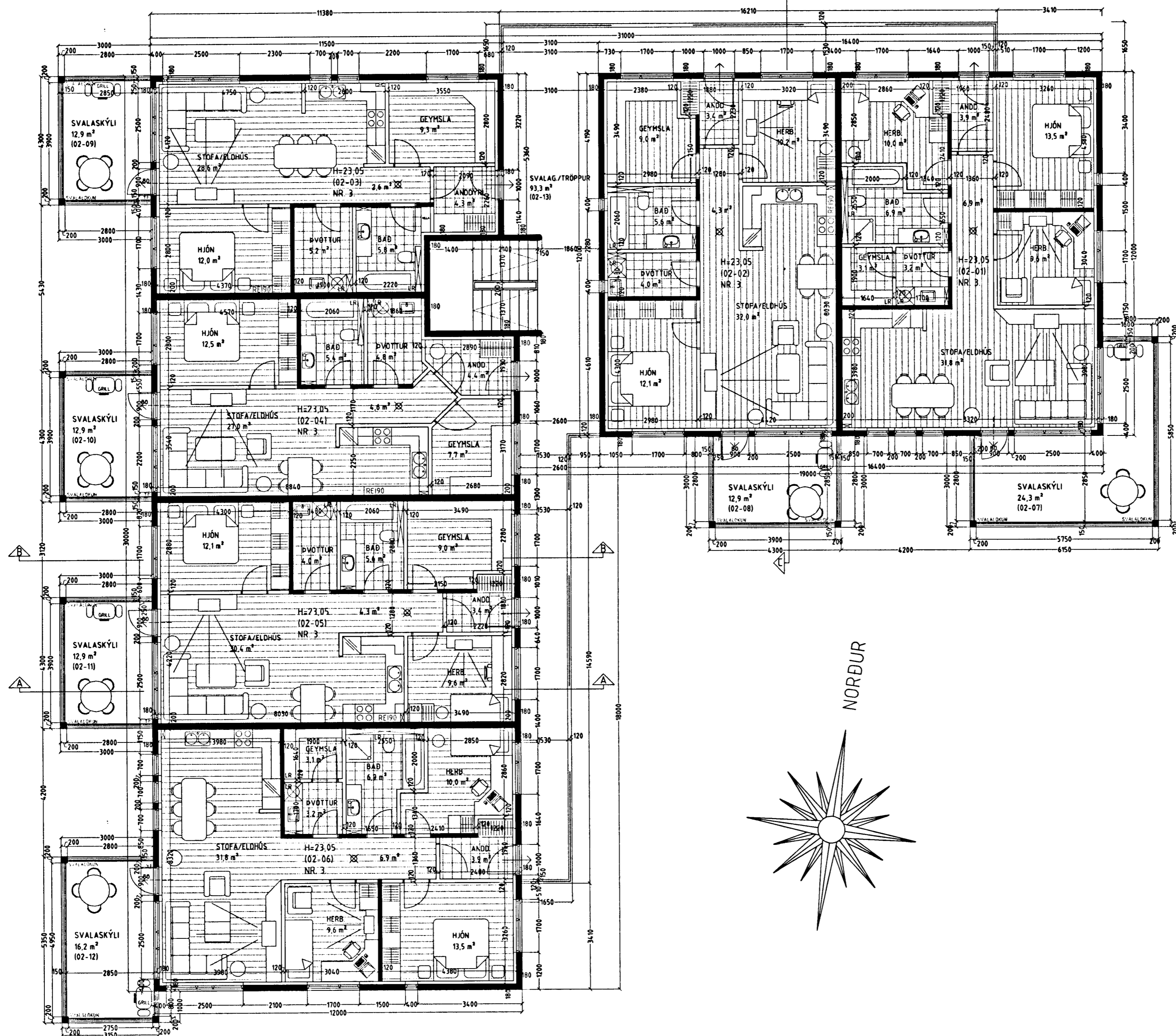
GRUNNMYND 2. HÆÐ MKV. 1:100.
