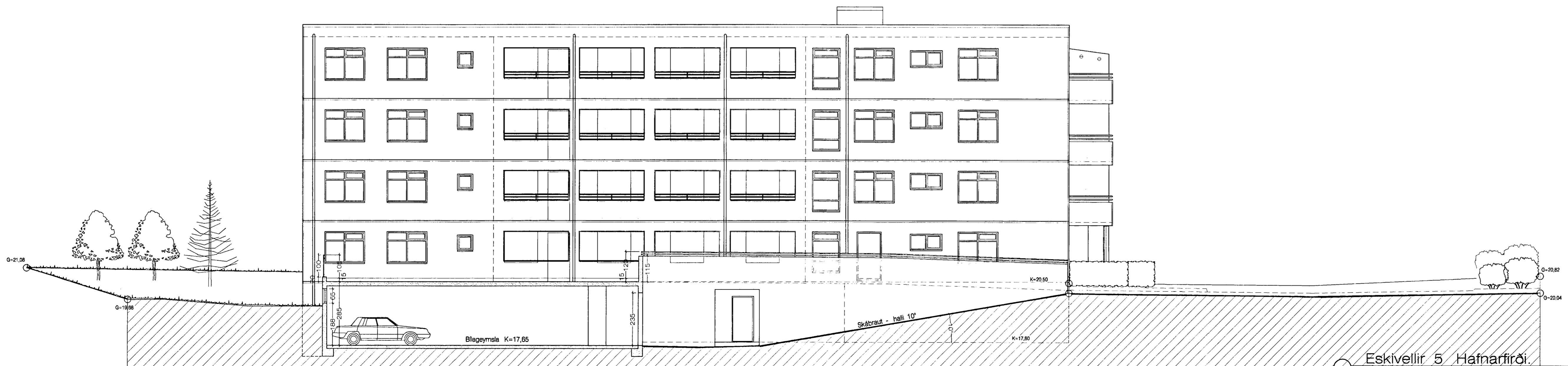
Norðurhlíð. 1:100 Sneiðing í Bílgeymslu.
