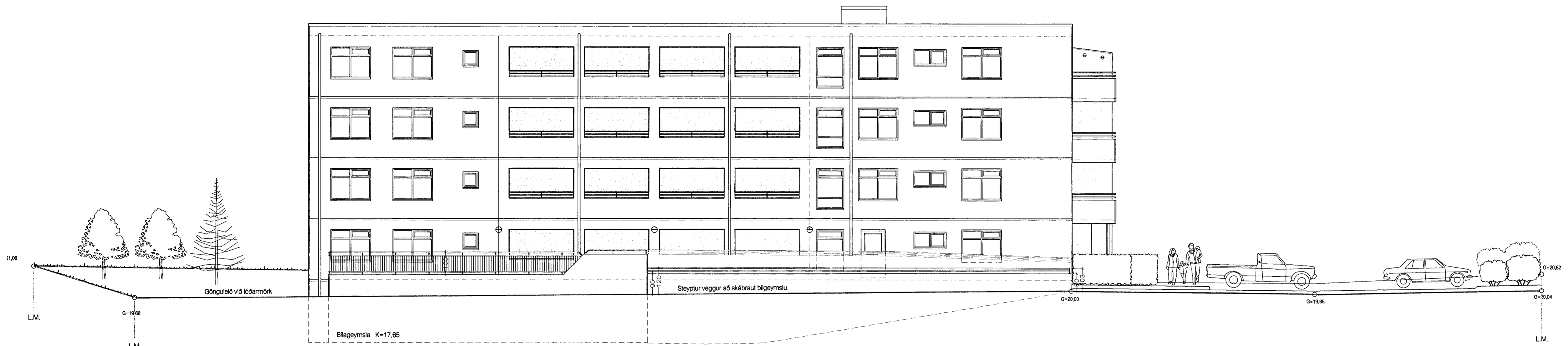
Norðurhlíð. 1:100
