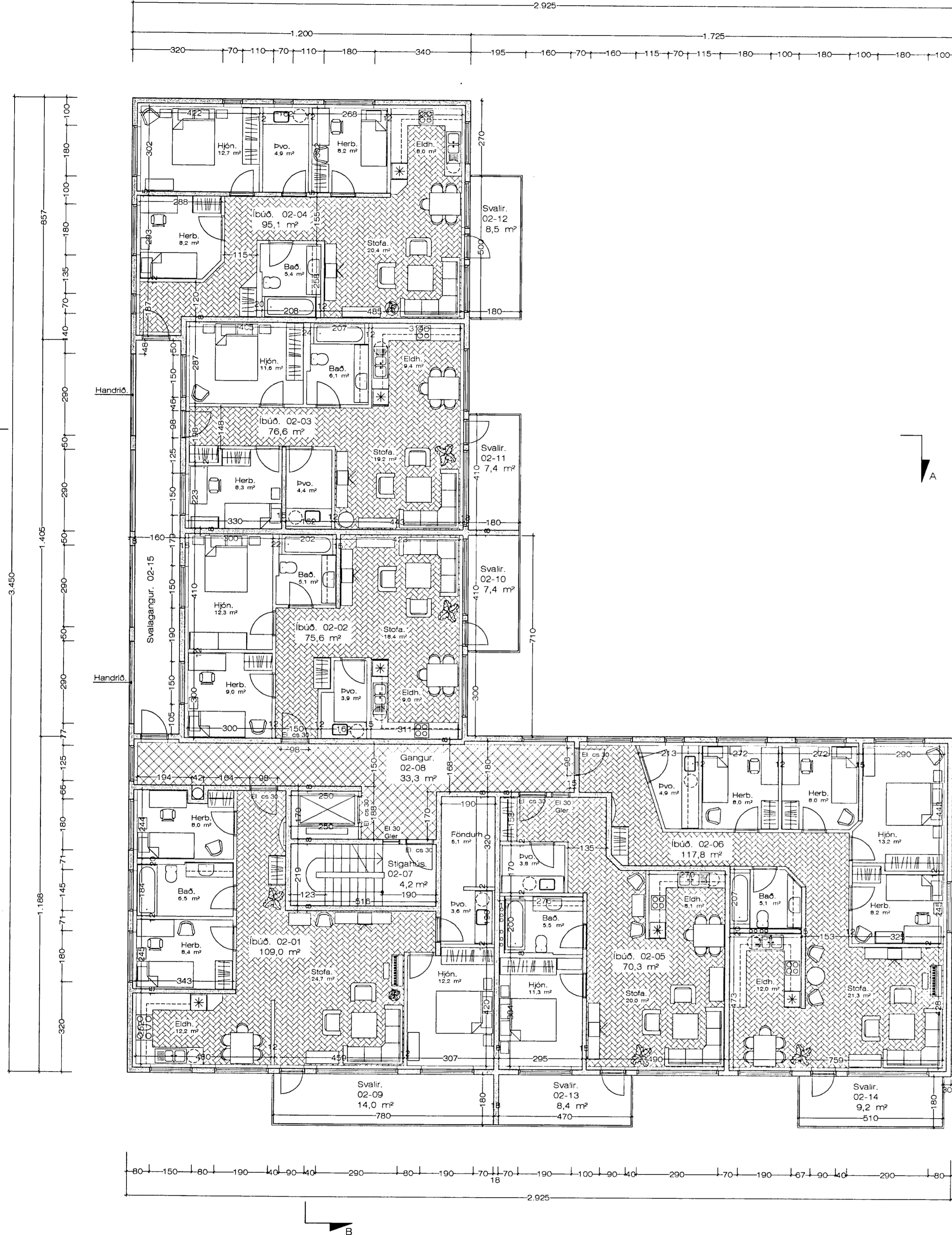
Grunnmynd. 2. og 3. hæð. 1:100 Stærð. 596,2 m 2
