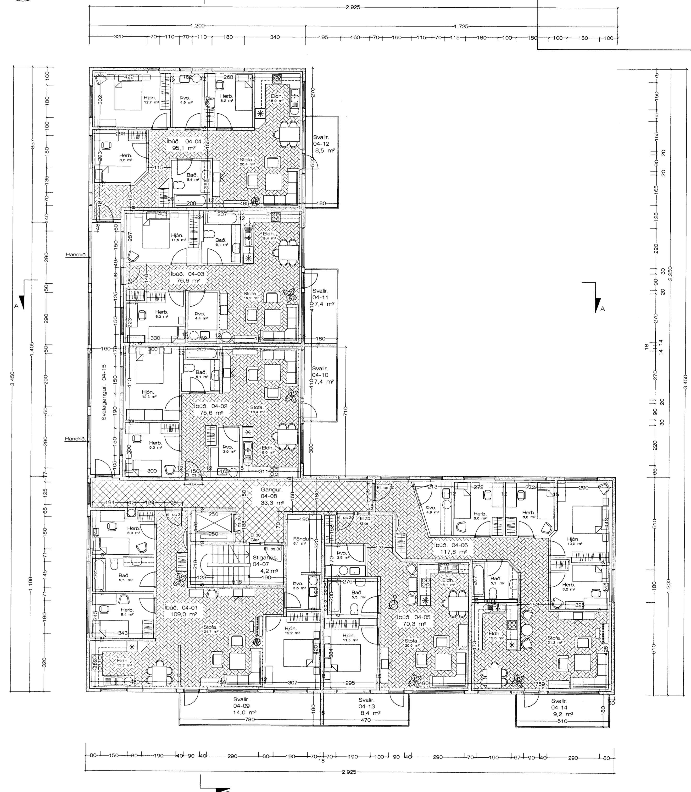
Grunnmynd. 4. hæðar. 1:100 Stærð. 596,2 m 2
