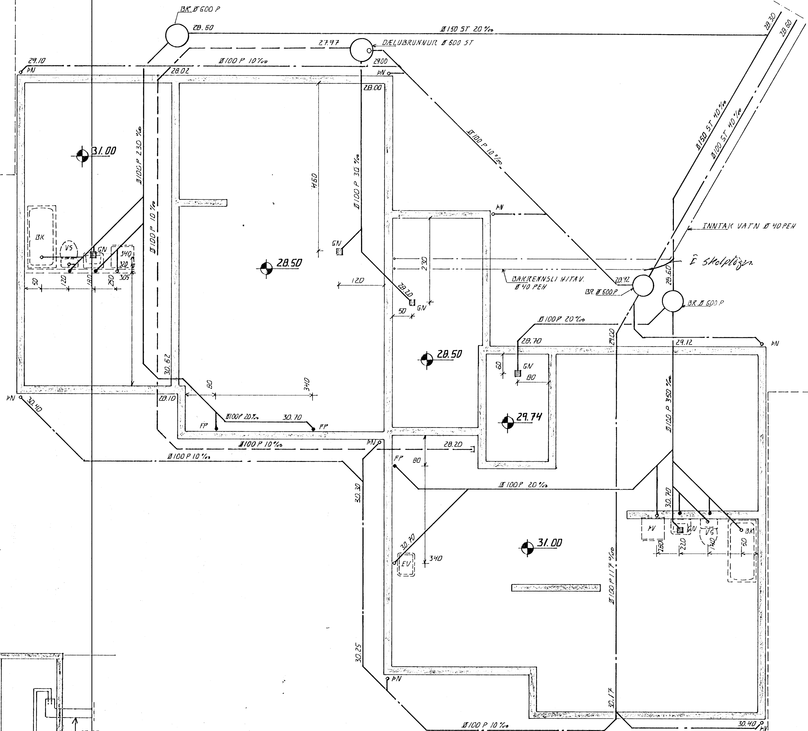
GRUNNMÝND, 1:50
