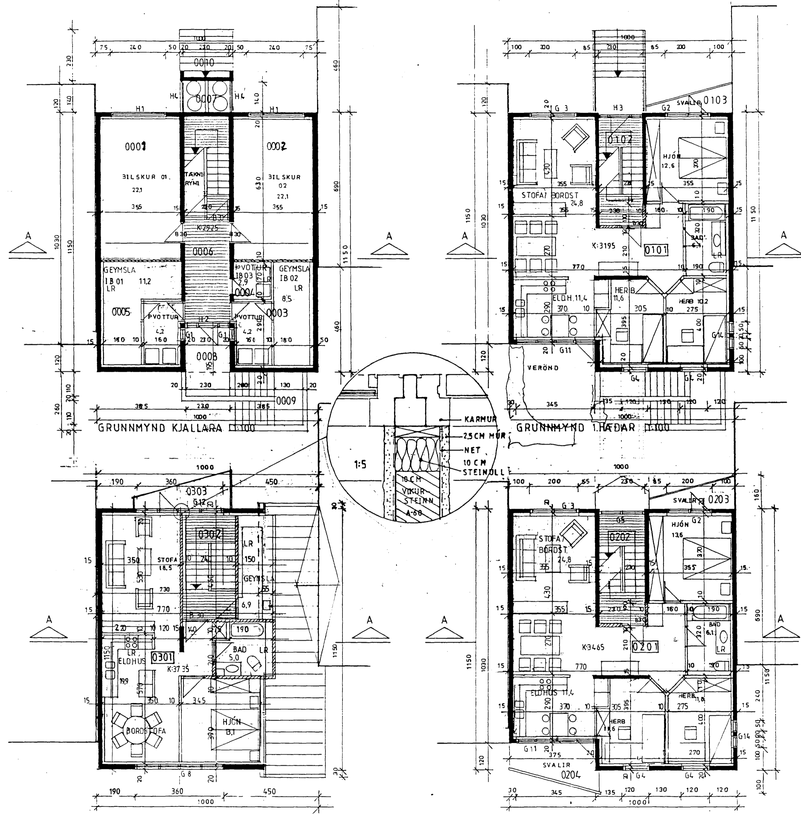
GRUNNMYND RISHÆÐAR 1:100
