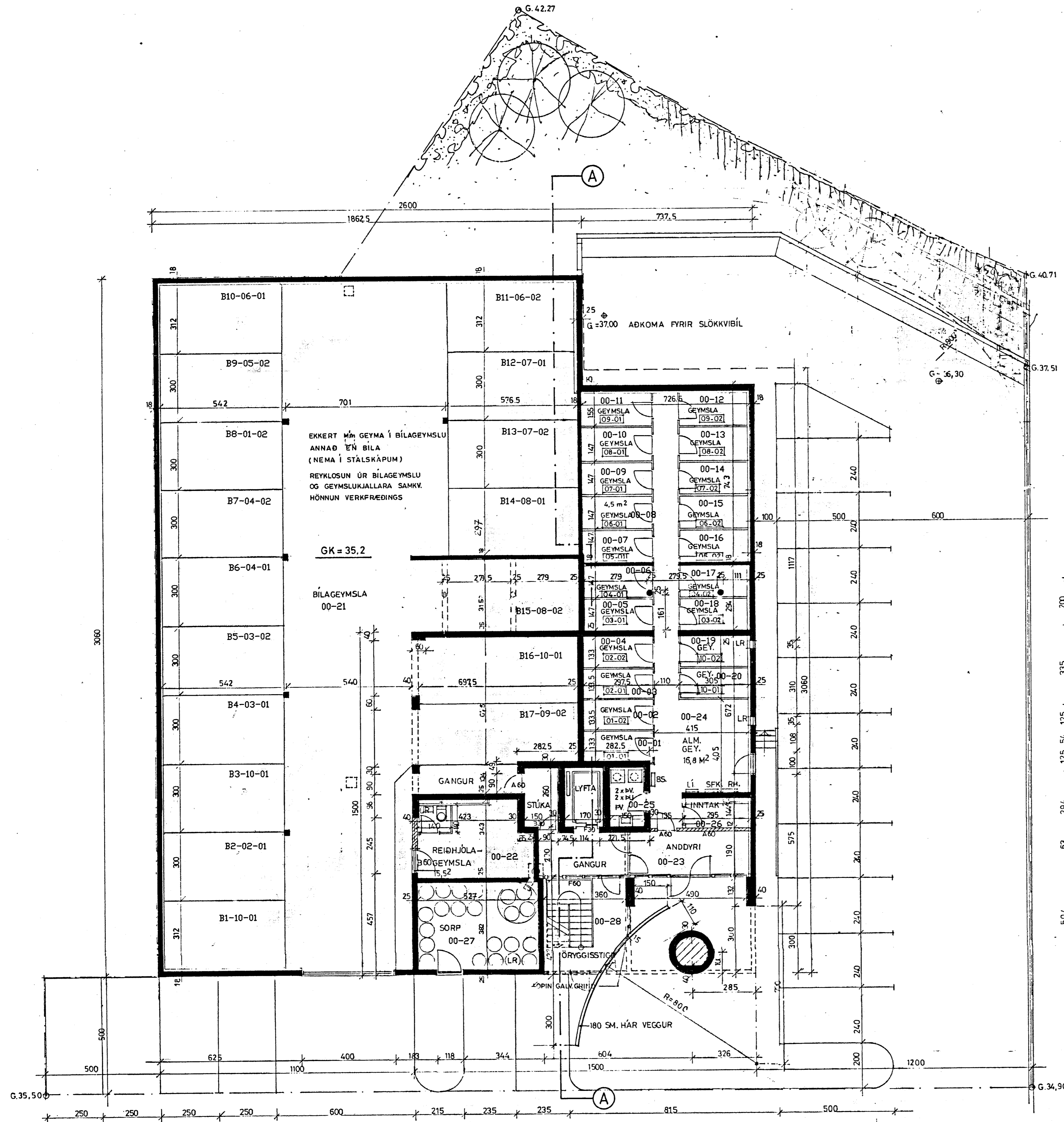
GRUNNMYND 00 1:100
