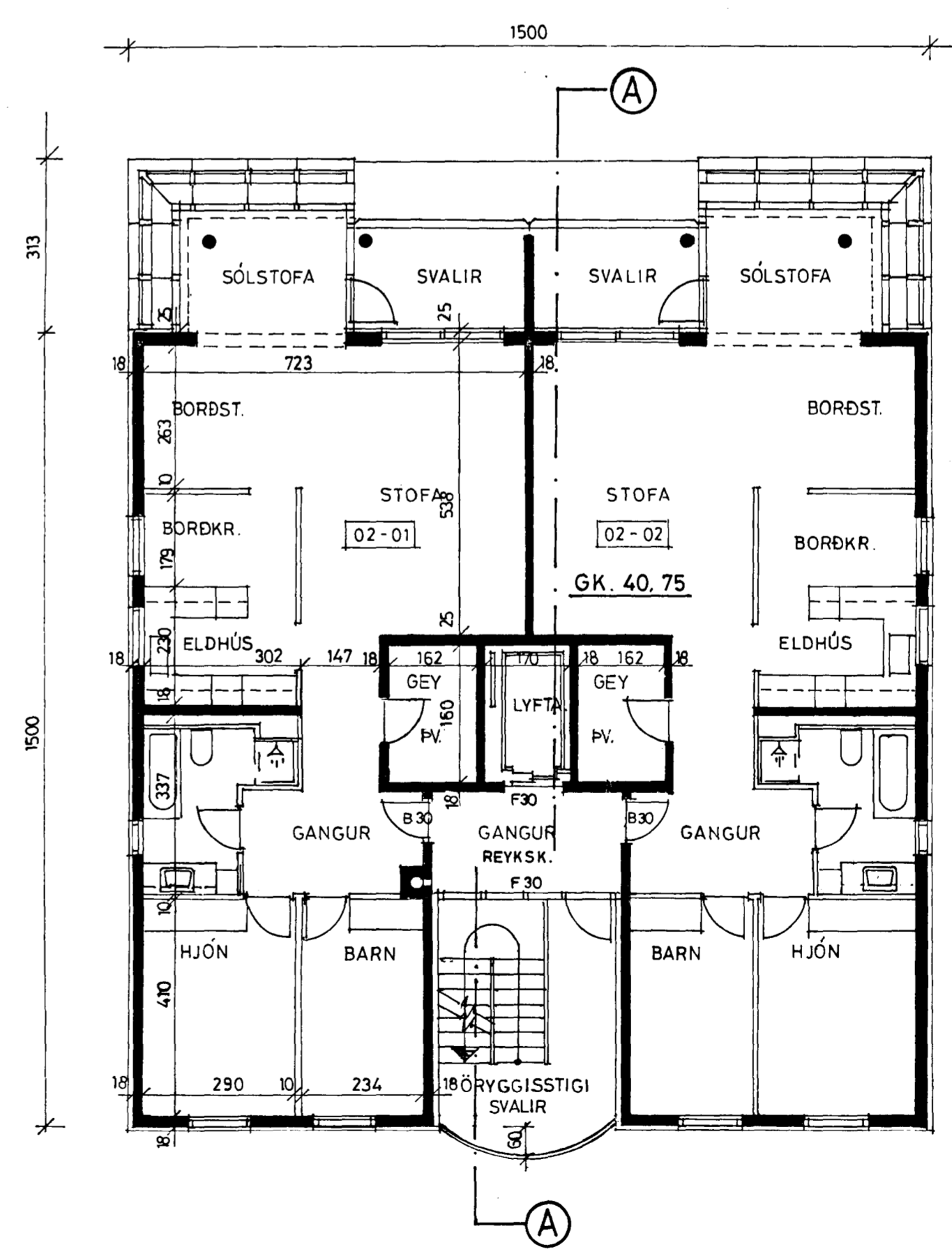
GRUNNMYND 02 1:100
