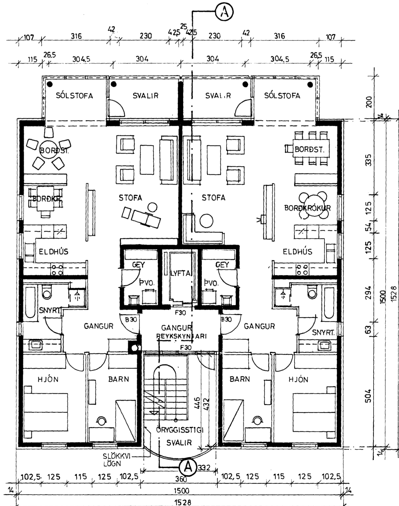
GRUNNMYND 03 - 09 1:100
