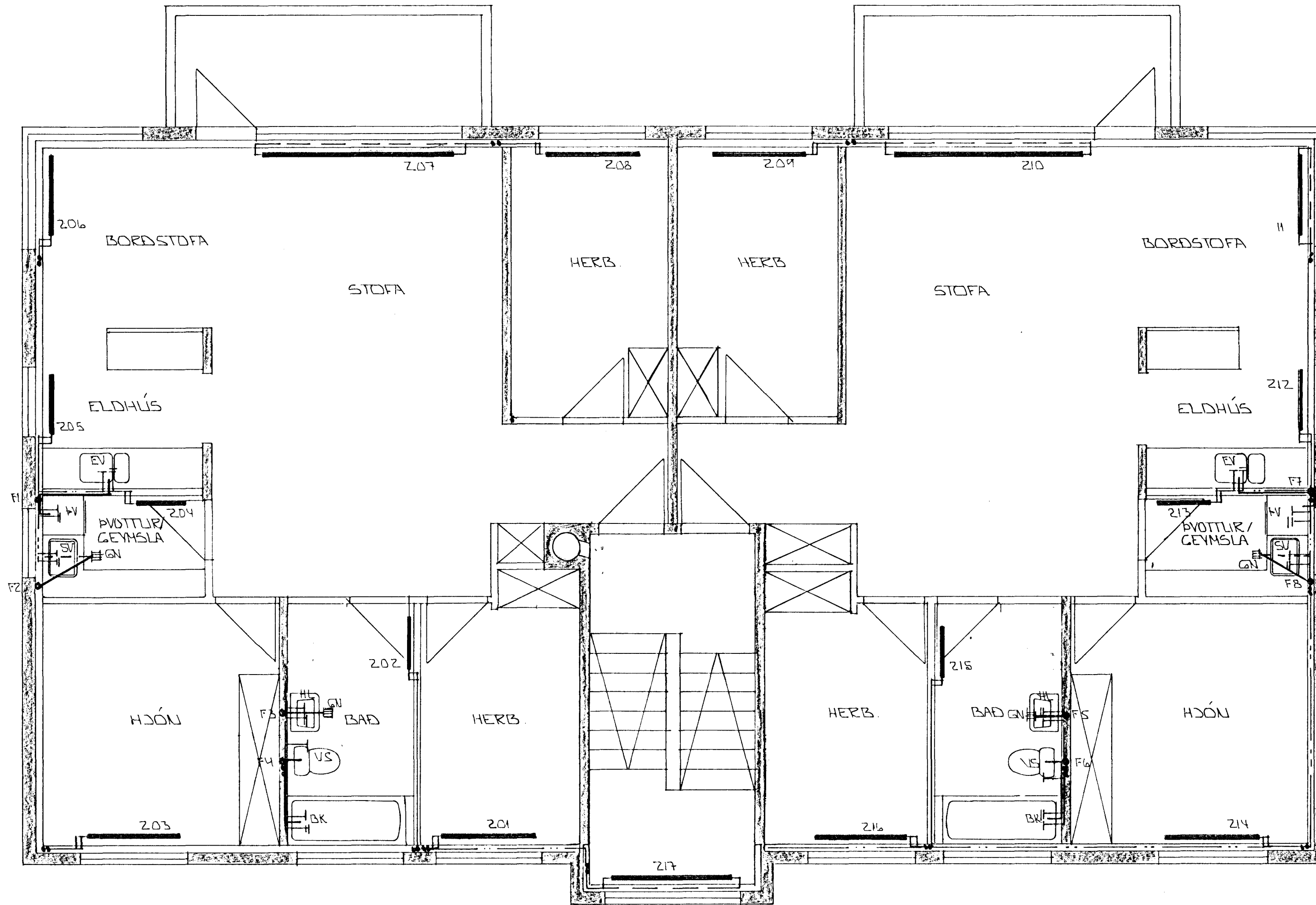
GRUNNMYND 2. HÆÐ 1:50
