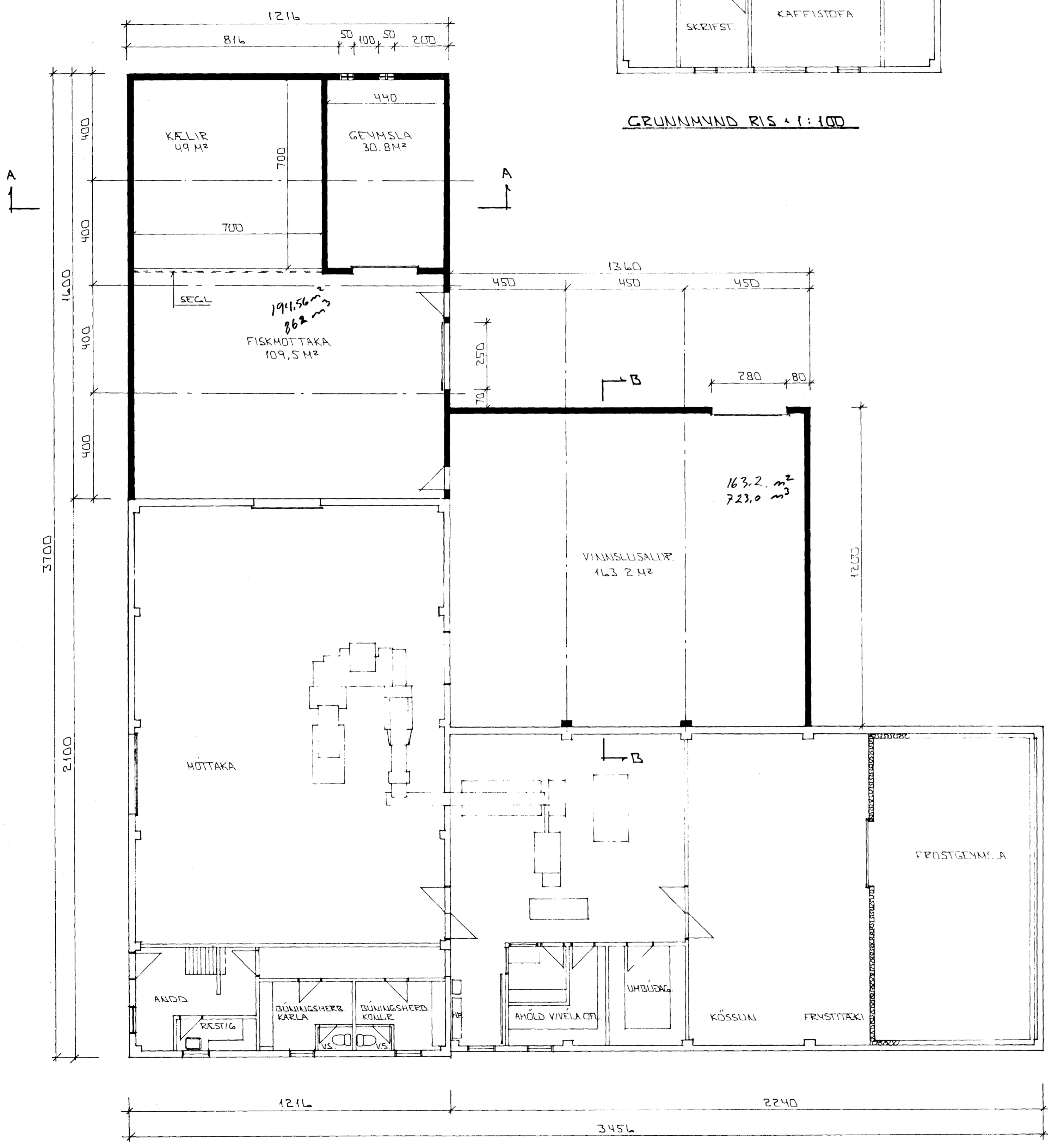
GRUNNMÝND + 1:100
