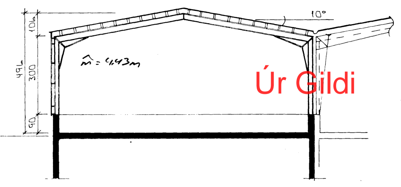
SNID B-B + 1:100
