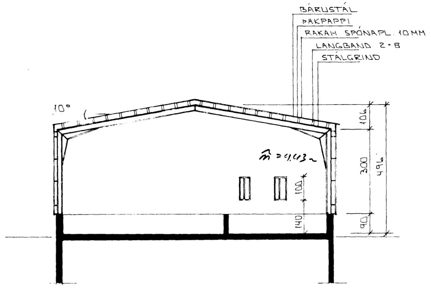
SNID A-A + 1:100
