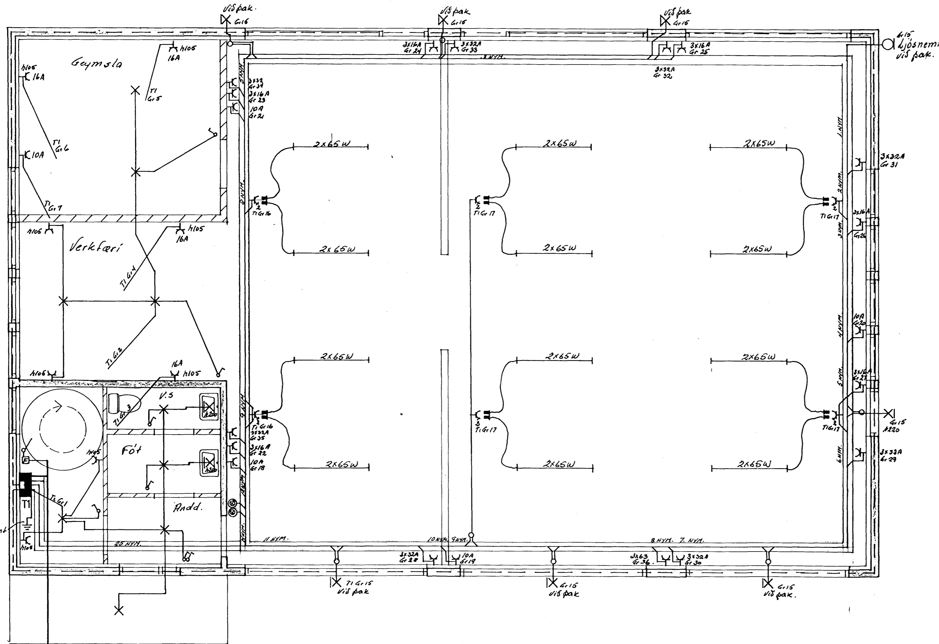
GRUNNMYND M 1:50
