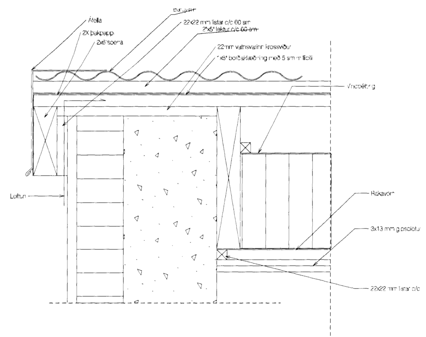
Deili 2 frágangur við gaff
