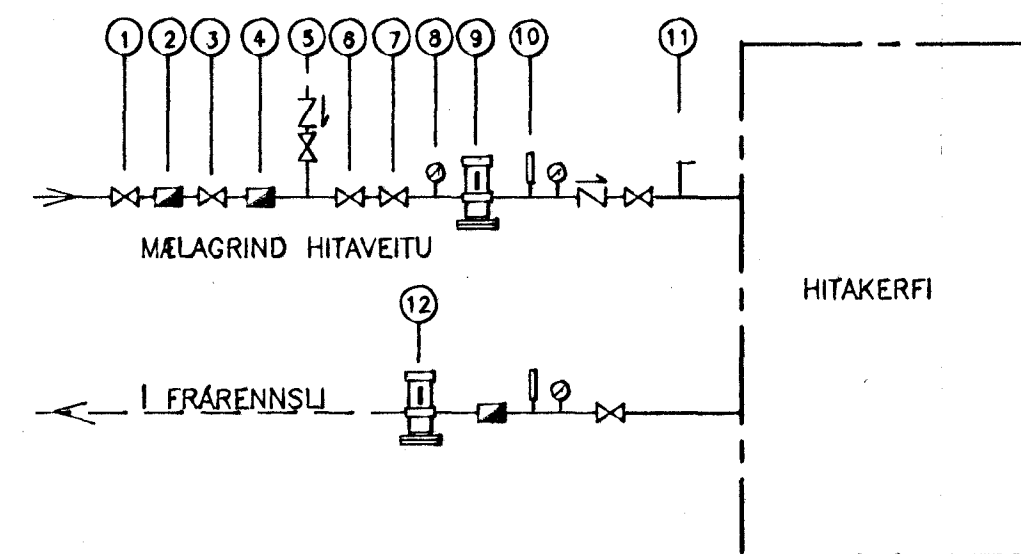
TENGIGRIND 1:20
