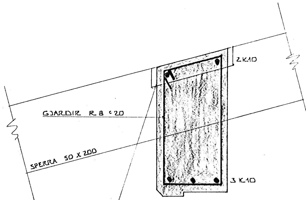
DEILI L ~ 1:5 TEIKN 1-09
