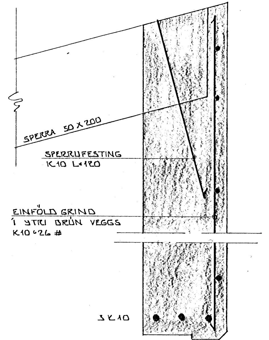
DEILI N ~ 1:5 TEIKN 1-09
